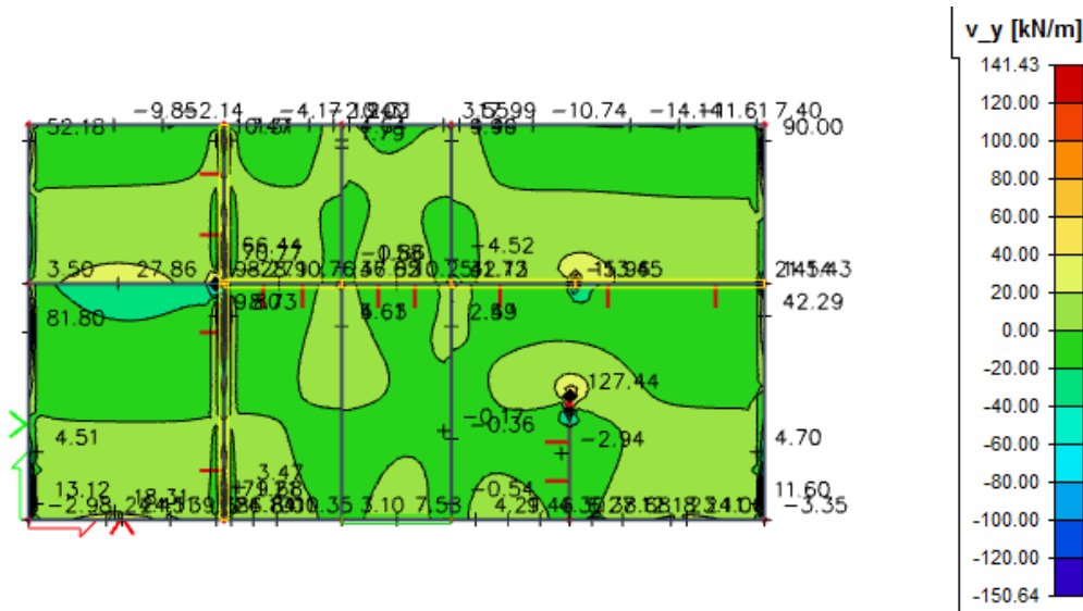
Slika 7.8 Poprečne sile V_{Ed,y} (kN/m) za GSN-1
