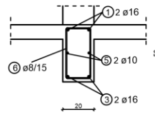
Presjek 1-1 MJ 1:25
