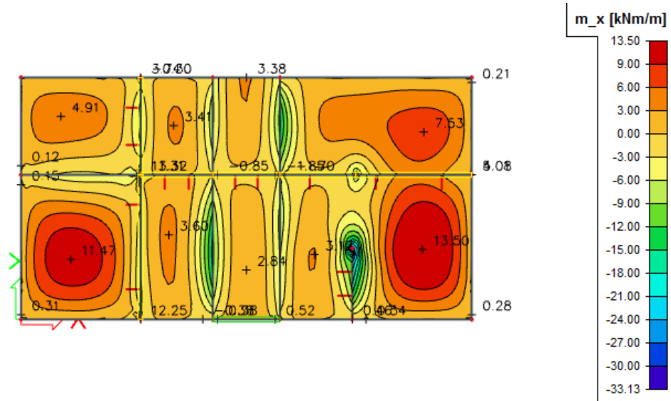
Slika 7.2 Moment savijanja (polje) M_{Ed,x} (kNm/m) za GSN
