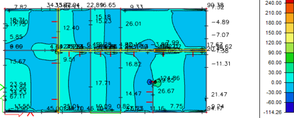
Slika 7.7 Poprečne sile V_{Ed,x} (kN/m) za GSN-1
