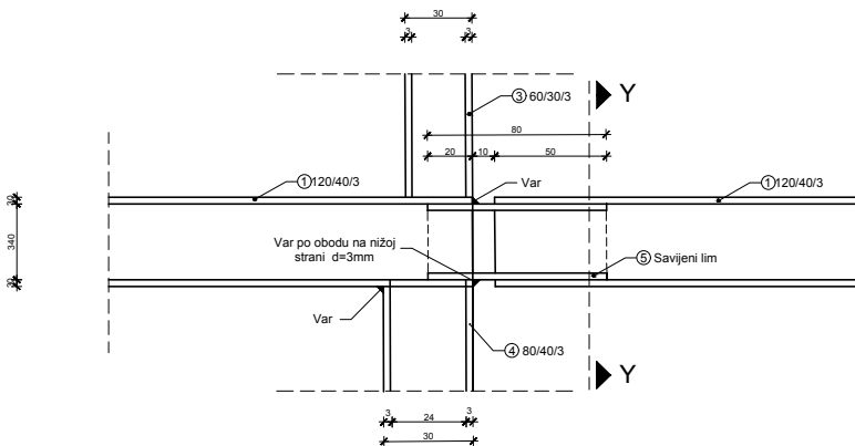
Detalj D 2 1:2
