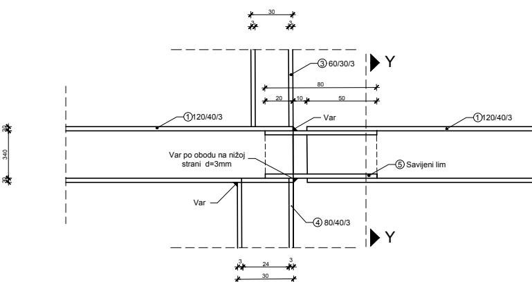
Detalj D 2 1:2
