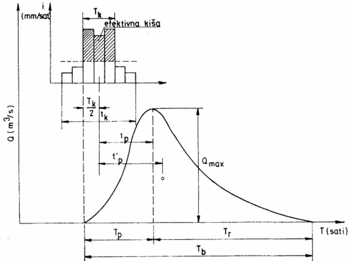
Slika 3: hidrogram (1)
