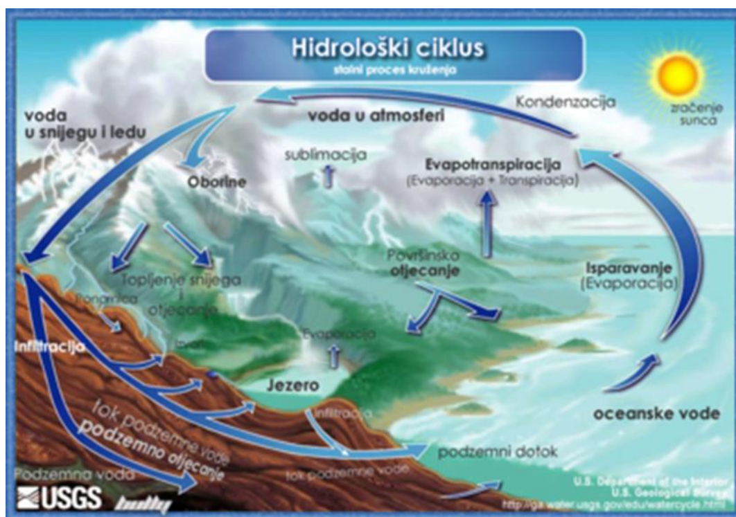
Slika 1. : Hidrološki ciklus [9]
