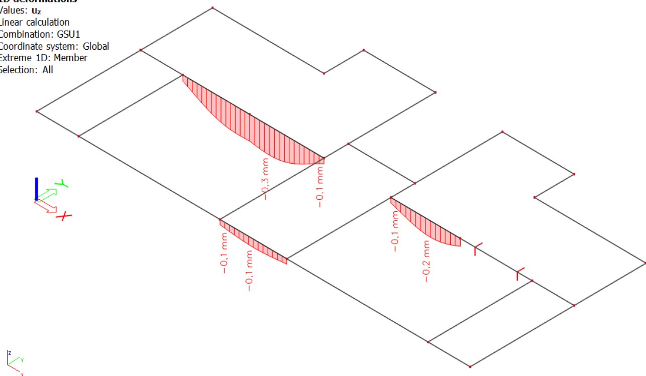
Slika 8.7 Progib grede (mm) za kombinaciju GSU-1
