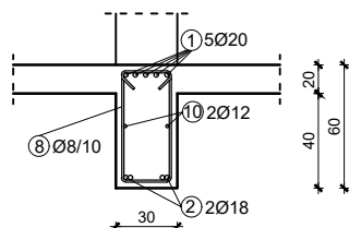
Presjek 4-4 (M 1:25)
