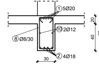
Presjek 3-3 (M 1:25)
