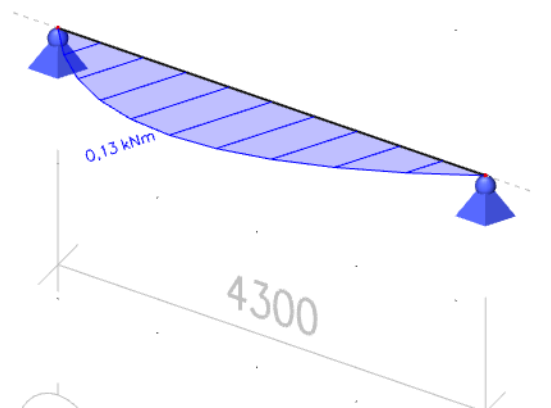
Slika 32 Dijagram momenata M_y i M_z za kombinaciju 4
