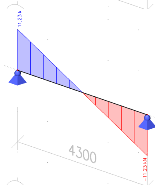
Slika 31 Dijagram poprečnih sila V_y i V_z za kombinaciju 3
