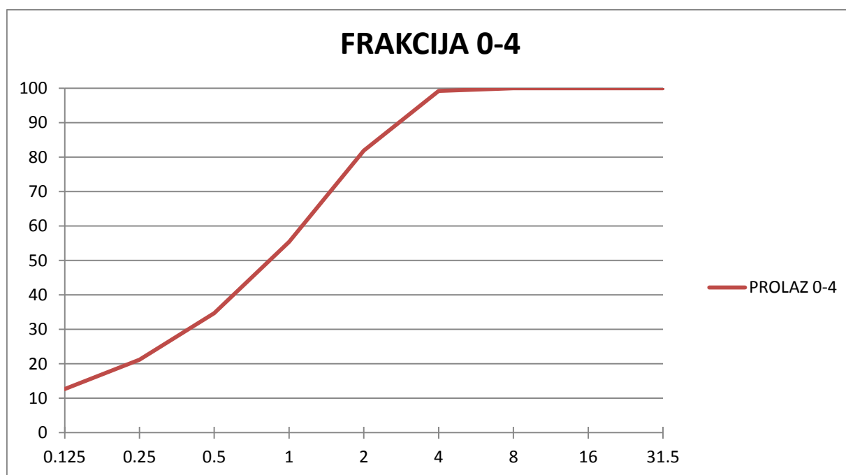
Slika 8.1. Granulometrijska krivulja agregata frakcije 0-4 mm
