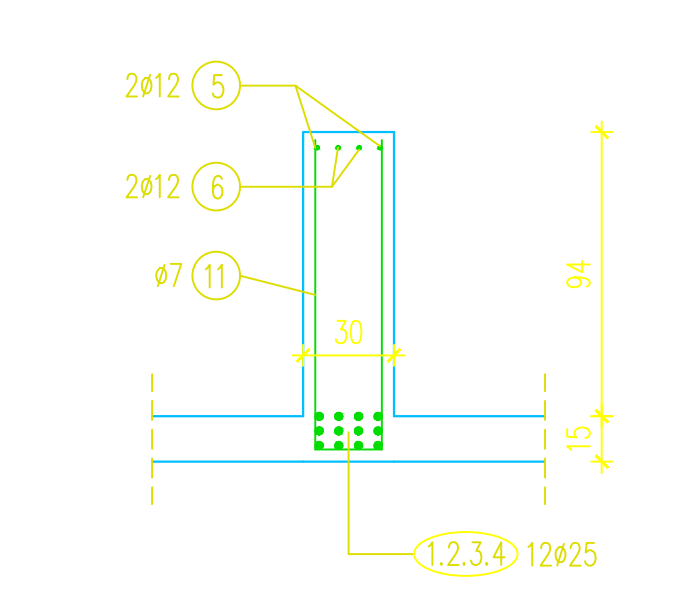
PRESJEK 3-3
