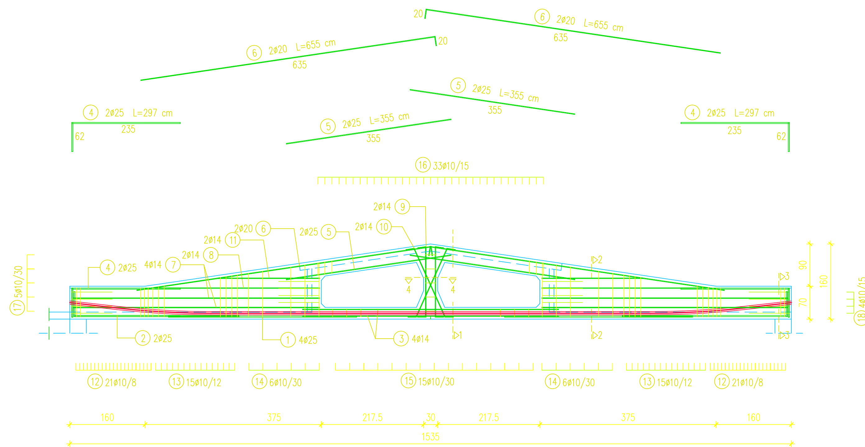
M=1cm:500kN
