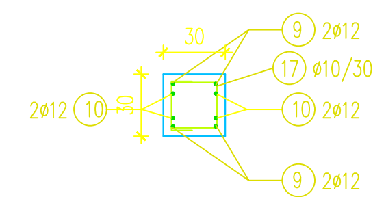
PRESJEK 4-4
