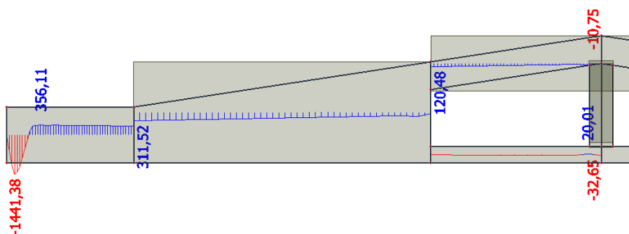
Slika 43. Dijagram poprečnih sila Vierendeel-ove grede [kN]
