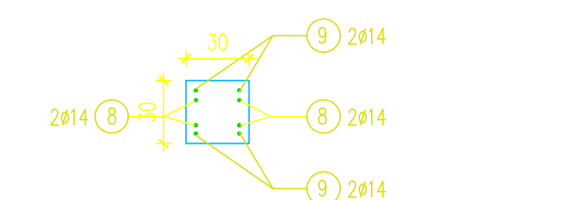
PRESJEK 6-6
