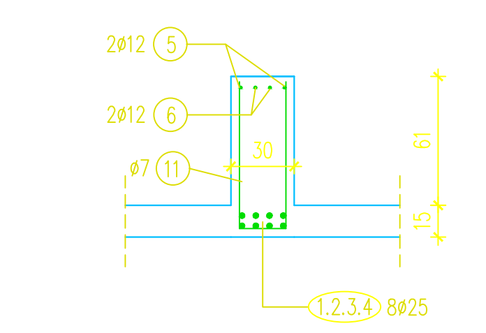
PRESJEK 4-4
