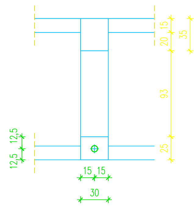
PRESJEK 10 – položaj kabela na sredini nosača
