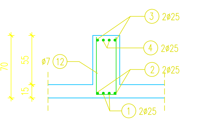
PRESJEK 5-5
