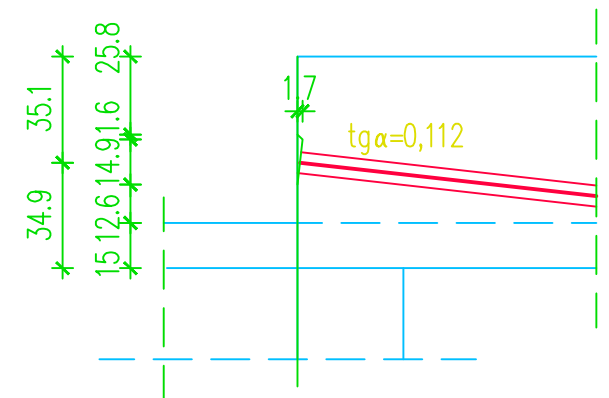
Detalj čela nosača
