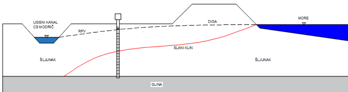
Slika 6.5. Položaj slanog klina u situaciji kada je voda u usisnom kanalu na niskoj koti, a razina mora na visokoj koti
