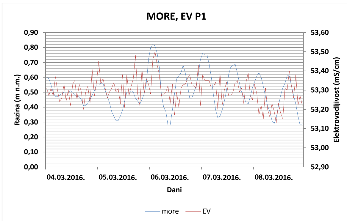
Slika 5.34. Grafički prikaz odnosa mora i elektrovođljivosti u P1 za razdoblje 04. – 08.03.2016.
