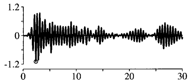
Slika 3 Akceleroگرام potresa 3
