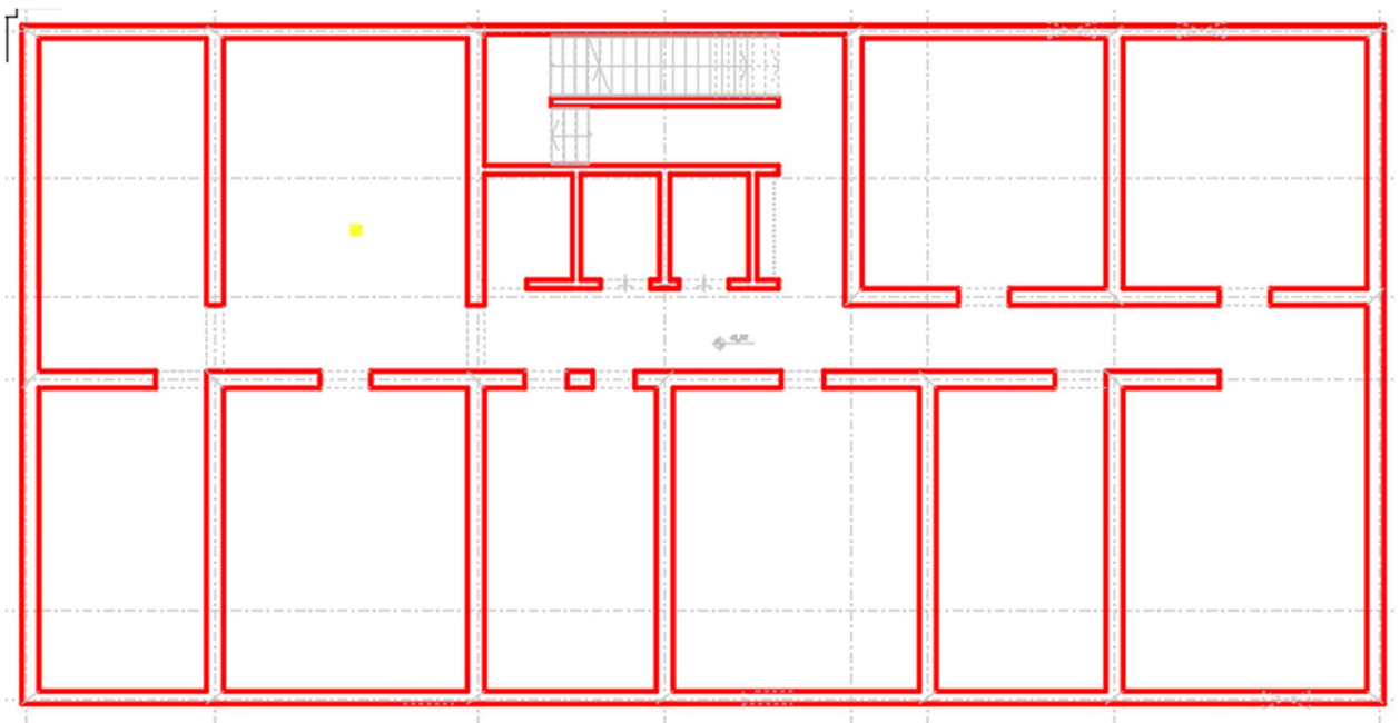
Slika 2.4. Sustav nosivih zidova etaže -1
