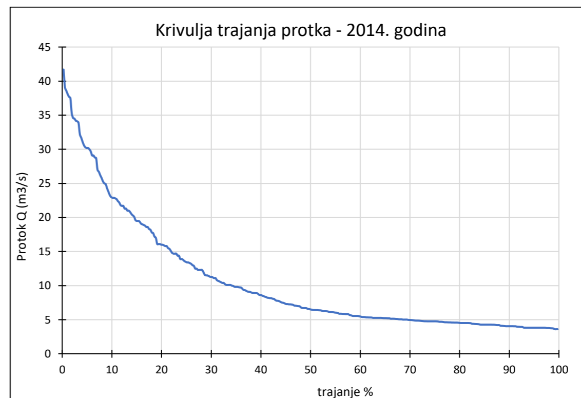
Graf 42. Krivulja trajanja protoka za 2014. godinu
