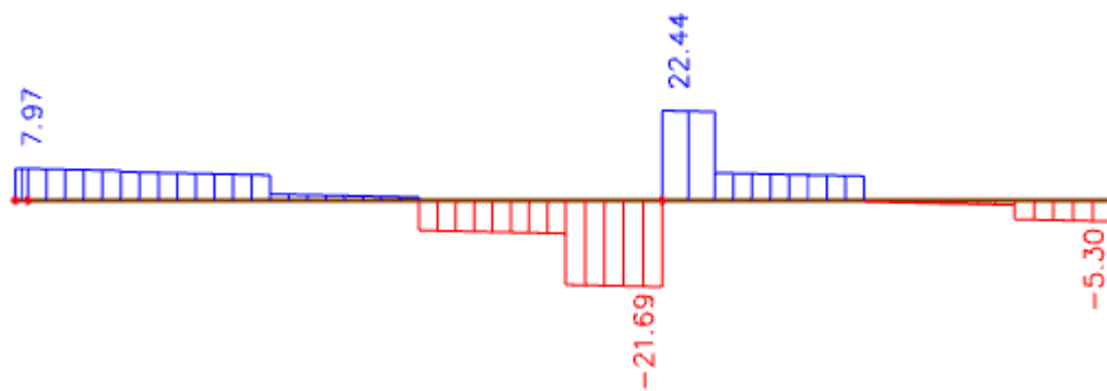
Slika 10.12 Poprečne sile V_z (kN)
