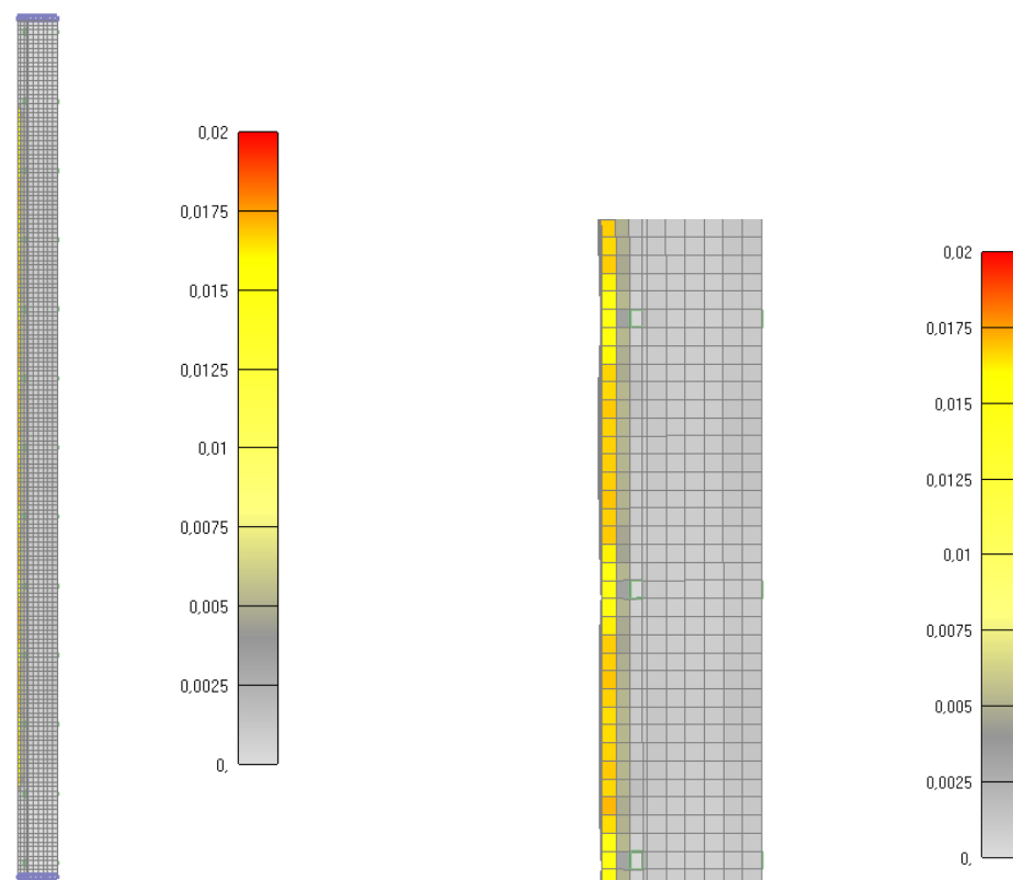
Slika 6.24: Prikaz pukotina za jednu četvrtinu stupa nakon 1615 minuta ( lijevo-cijeli stup, desno-detalj stupa )-KRAJ KONSTANTNOG HLADJENJA
