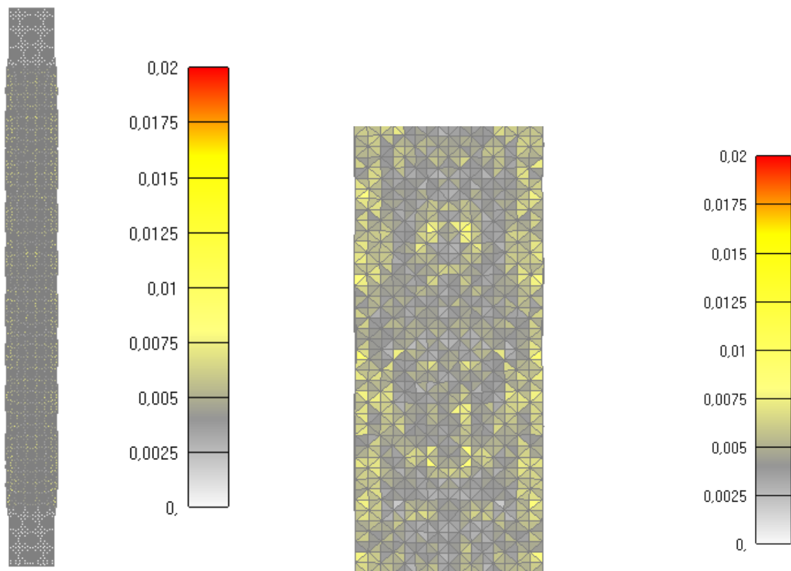
Slika 6.64: Prikaz pukotina za cijeli stup nakon 60 minuta ( lijevo-cijeli stup, desno-detalj stupa )
