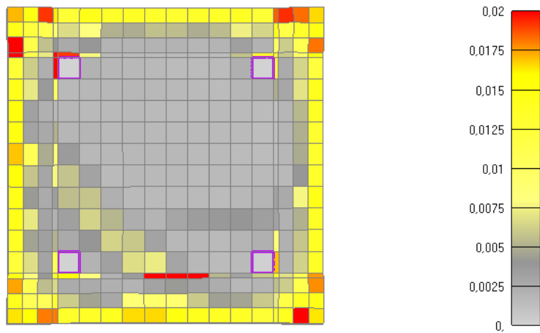
Slika 6.111: Prikaz pukotina za poprečni presjek stupa nakon 175 minuta požara (gore-sa sponama, dolje-bez spona)-KRAJ LINEARNOG I POČETAK KONSTANTNOG HLADENJA
