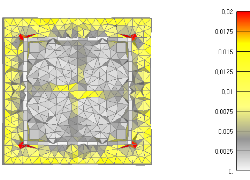
Slika 6.49: Prikaz pukotina za poprečni presjek stupa nakon 275 minuta požara (sa sponama)
