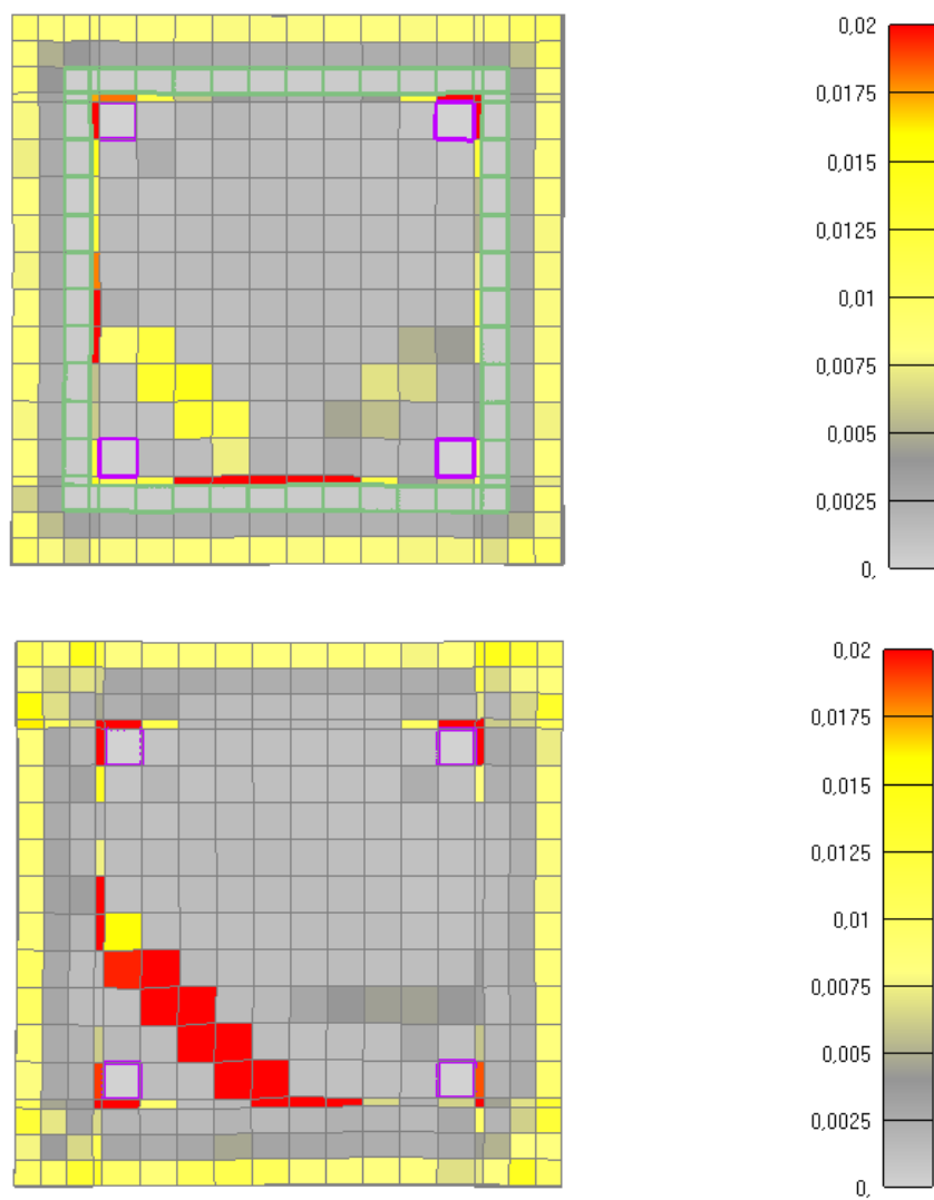
Slika 6.110: Prikaz pukotina za poprečni presjek stupa nakon 115 minuta požara (gore-sa sponama, dolje-bez spona)
