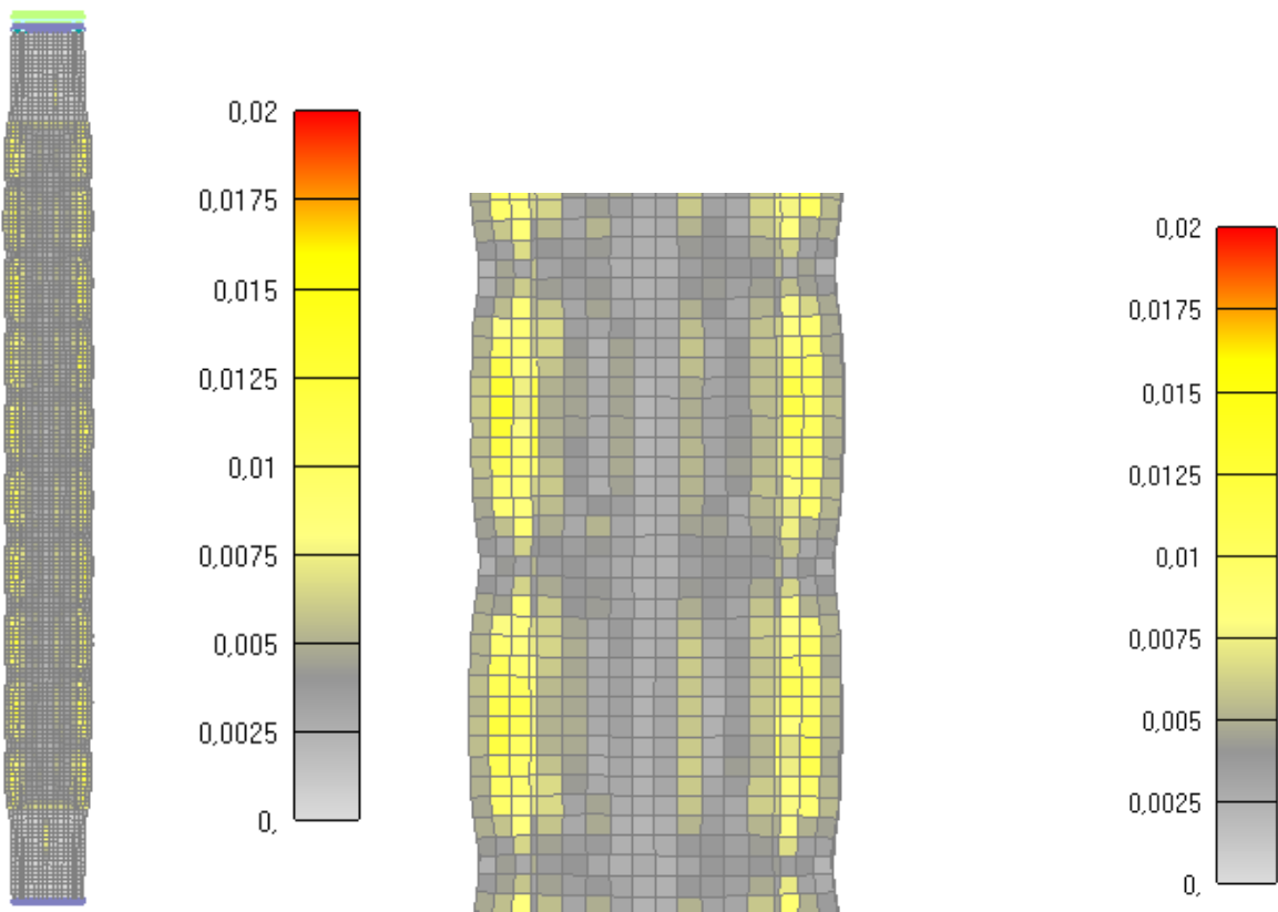
Slika 6.186: Prikaz pukotina za cijeli stup nakon 90 minuta (lijevo-cijeli stup, desno-detalj stupa) -KRAJ GRIJANJA I POČETAK HLAĐENJA
