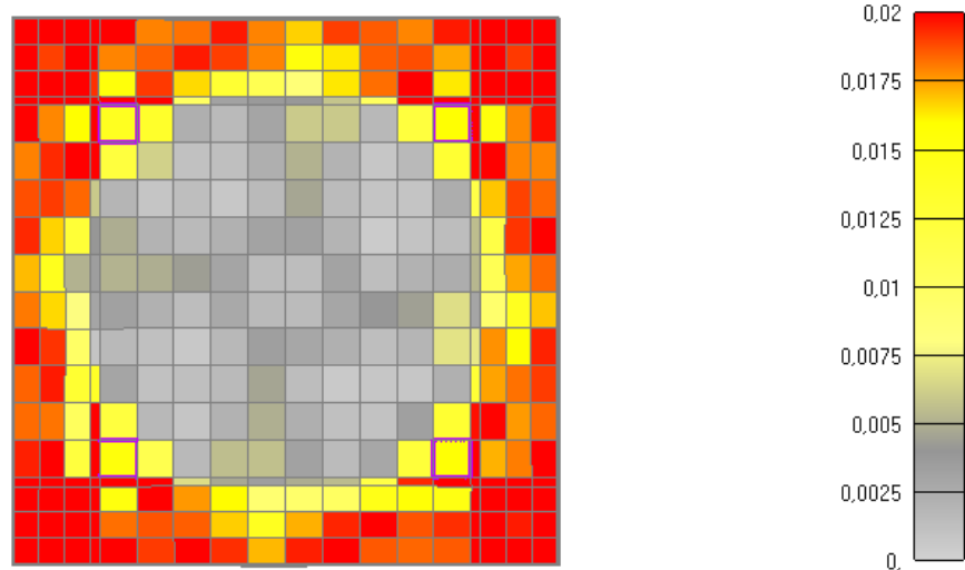
Slika 6.225: Prikaz pukotina za poprečni presjek stupa nakon 1090 minuta (gore-sa sponama, dolje-bez spona)
