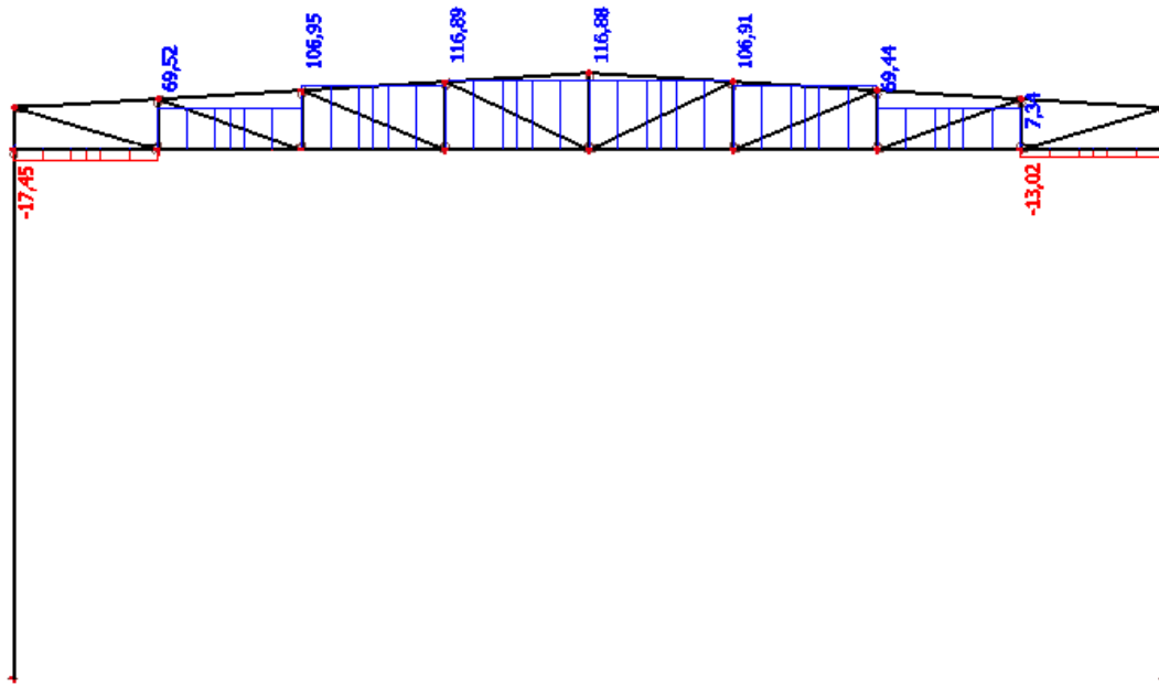
Slika 5.1.2.2. Maksimalna tlačna uzdužna sila u donjem pojasu rešetke
