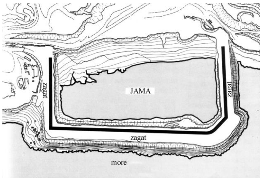
Slika 8.77 Tlocrt građevne jame zagata s fotografije 1.9 (Martin, 1980.)
