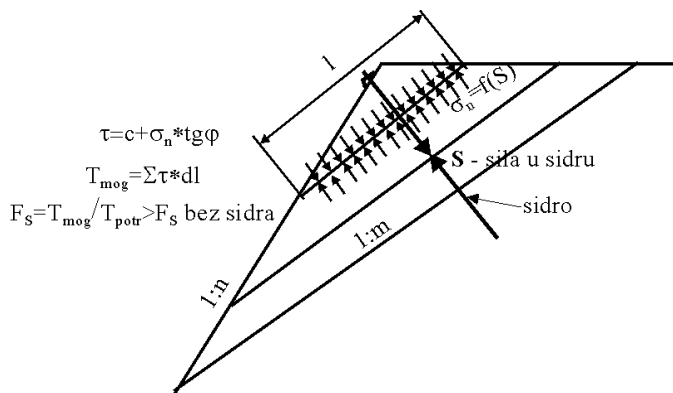
Slika 7.7 Utjecaj prednapetog sidra na blok koji «visi»
