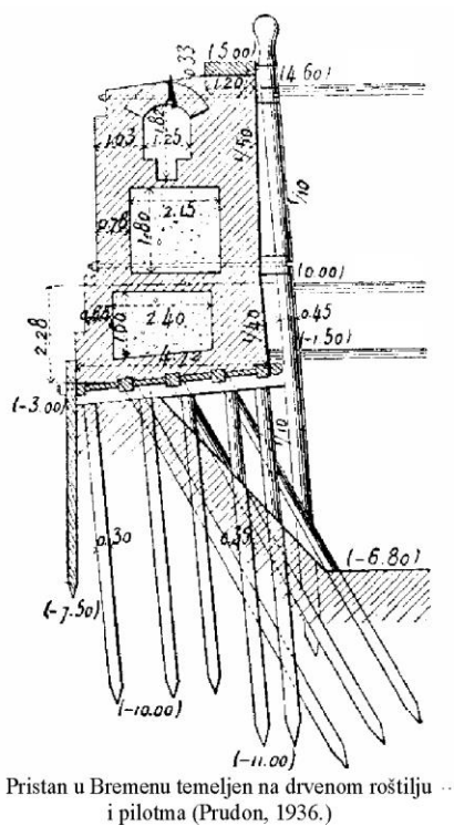
Slika 3.2 Masivni, gravitacijski potporni zidovi na dubokim temeljima
