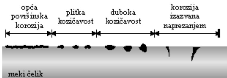
Slika 7.144 Vrste korozije na čeličnoj šipci
