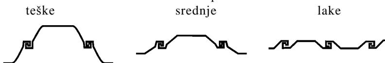
Slika 5.21 b: tip Larsen
