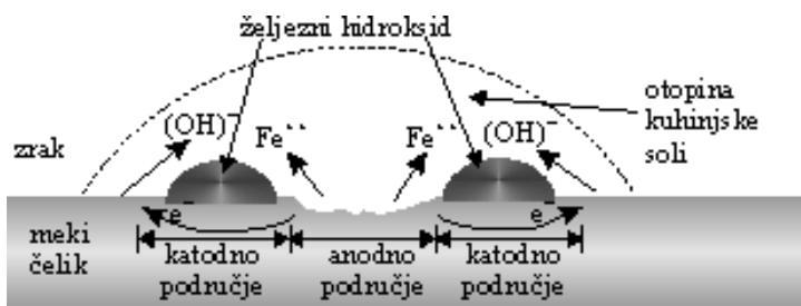
Slika 7.23 Idealizirana galvanska korozija (Hanna, 1982.)
