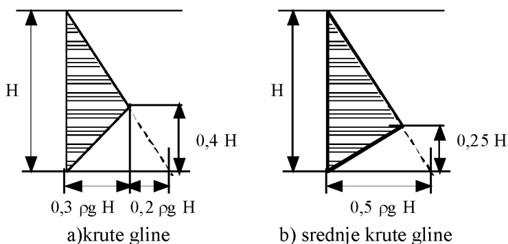
Slika 5.6 Raspodjela pritisaka (Tschebotarioff, 1973.)
