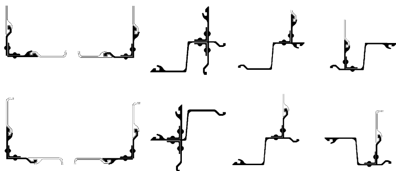
Slika 5.21 Poprečni presjeci čeličnih platica
