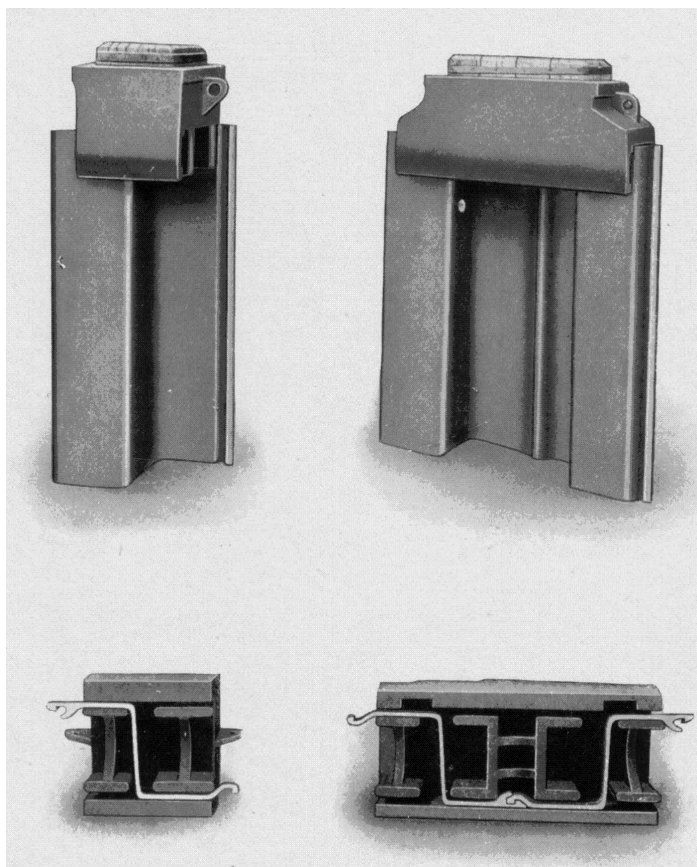
Slika 5.24 Posebni nastavci za zabijanje plaica (Hoesch-Kölnneussen, 1937.)
