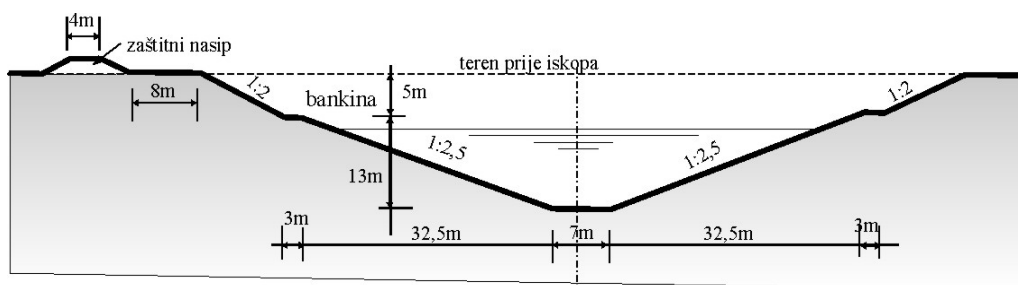
Slika 12.14 HE Varaždin, odvodni kanal ukopan u kvartarni nanos dravske terase Odteretni kanal Odra, služi za odvođenje velikih voda Save u Lonjsko polje.
