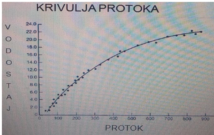
Slika 16. Krivulja protoka
