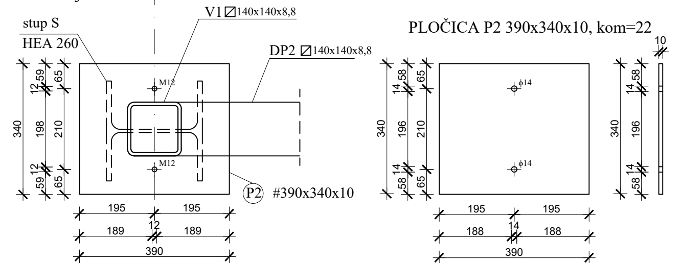
Presjek 2-2
