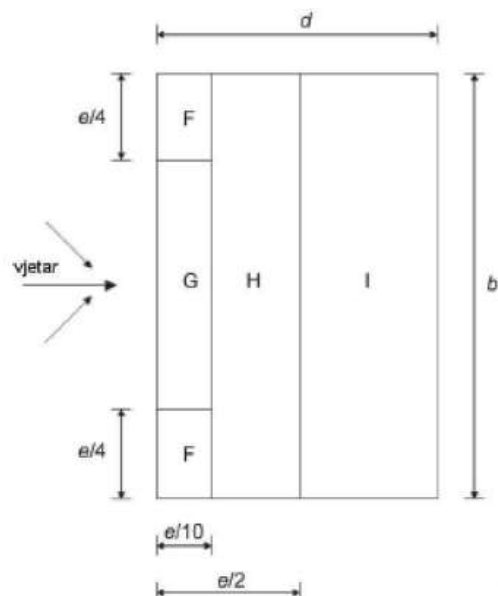
Slika 2.3. Prikaz područja vjetra za kose krovove
