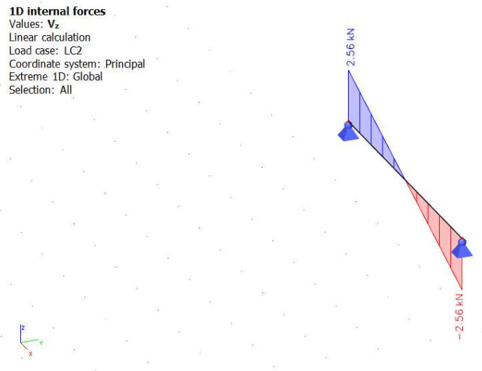
Slika 4.21. Dijagram poprečnih sila bočne podružnice
