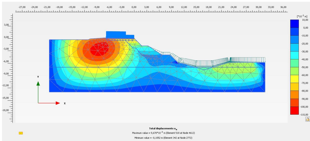
Slika 14. Ukupni pomaci uslijed potresa u smjeru x
