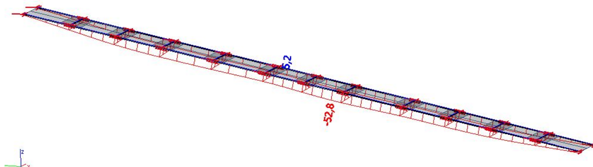
Slika 5.21. Prikaz vertikalnog pomaka grednih nosača
