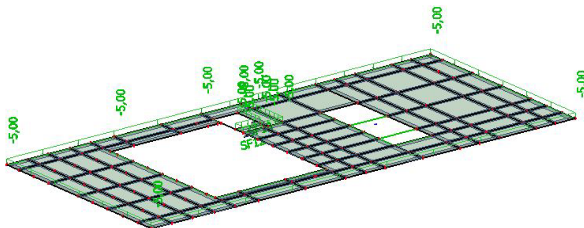
Slika 3.7. Prikaz raspodjele pokretnog opterećenja- ravni krov
