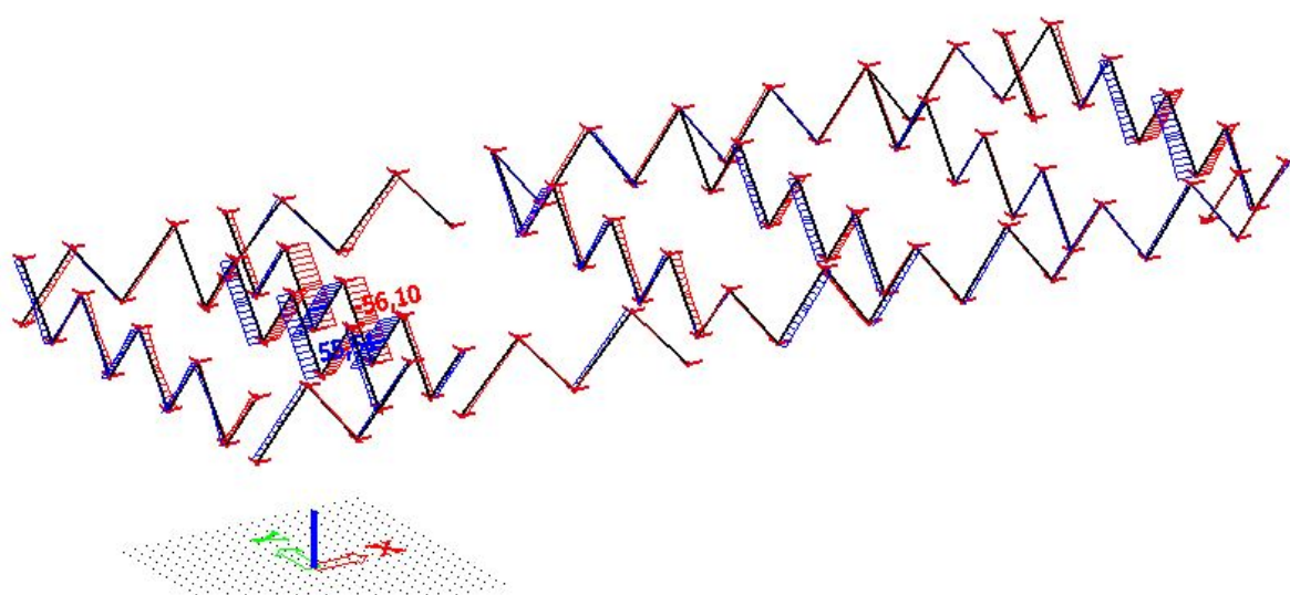
Slika 5.16. Rezne sile-Vy
