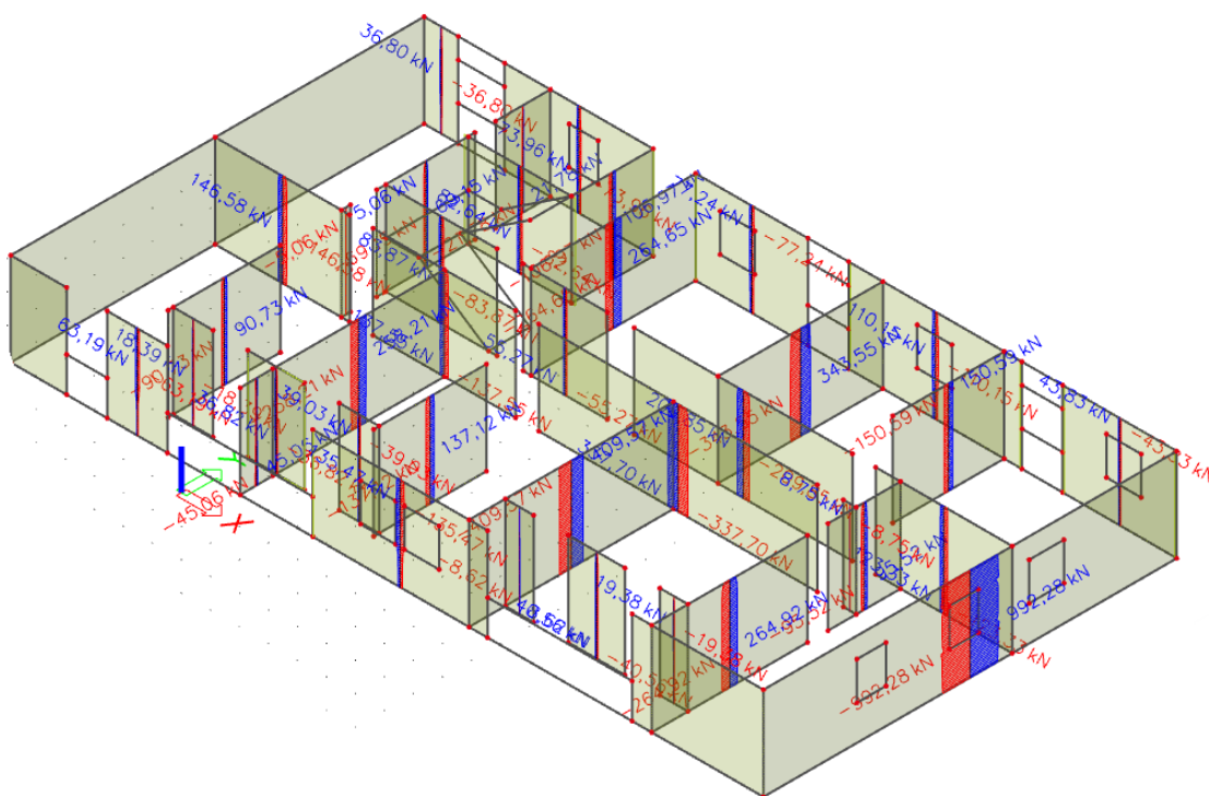
Slika 5.4: Dijagram poprečnih sila V [kN] za kombinaciju 1,32 S_y
