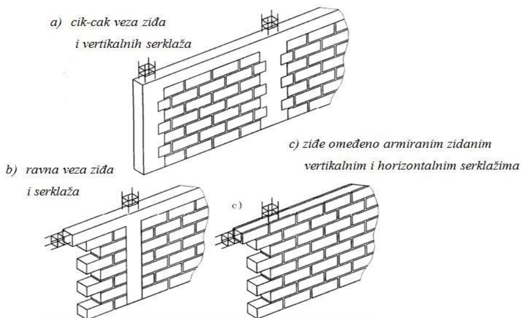
Slika 1.6: Primjeri omeđenog ziđa
