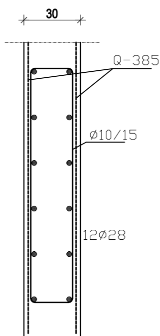
Detalj B
