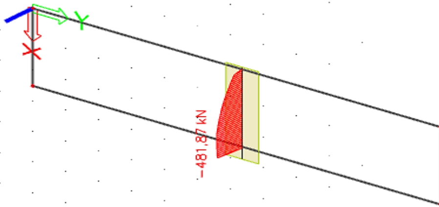
Slika 11.34. Maksimalna uzdužna sila za kombinaciju 1,35(g+dg)+1,5q+1,5(\rho_o+p_o)
