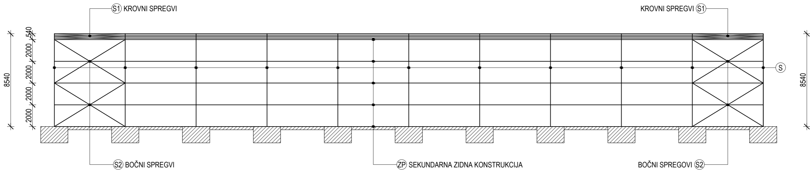
PRESJEK 2-2
