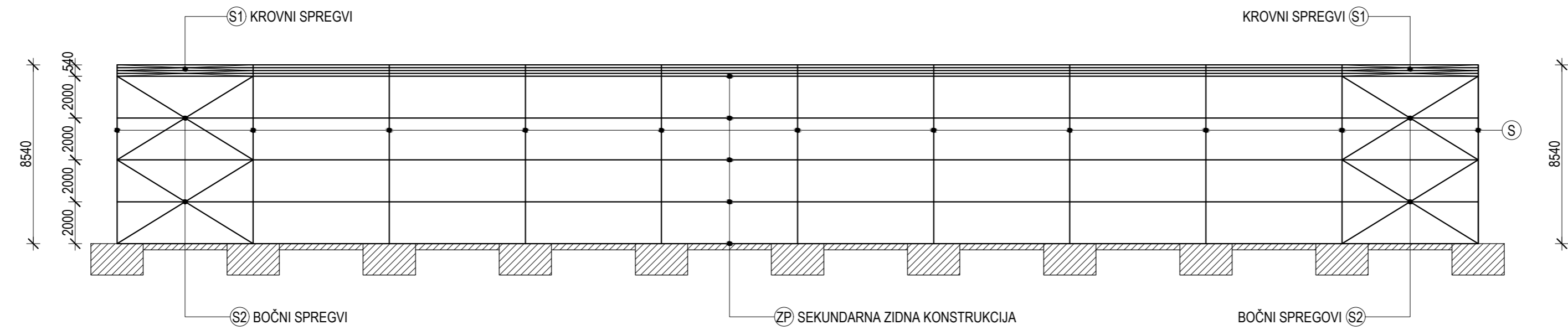
PRESJEK 2-2
