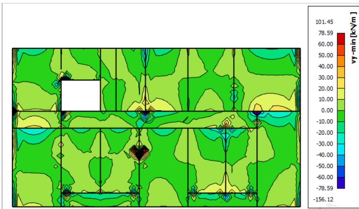
Slika 18. Poprečne sile V_{Ed,y} (kN/m) za GSN
