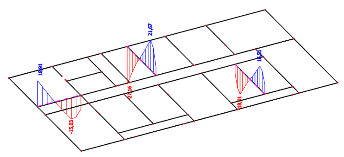
Slika 42. Poprečne sile V_z (kN) za GSN
