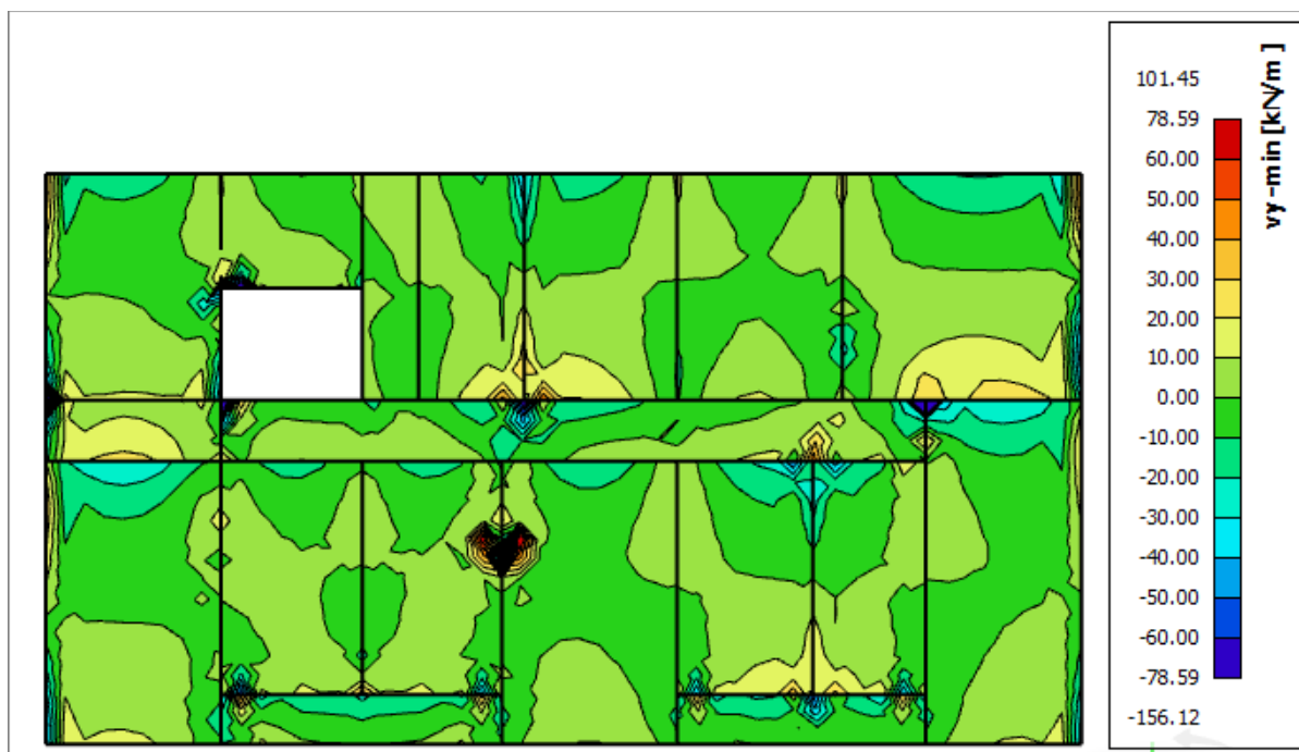
Slika 18. Poprečne sile V_{Ed,y} (kN/m) za GSN
