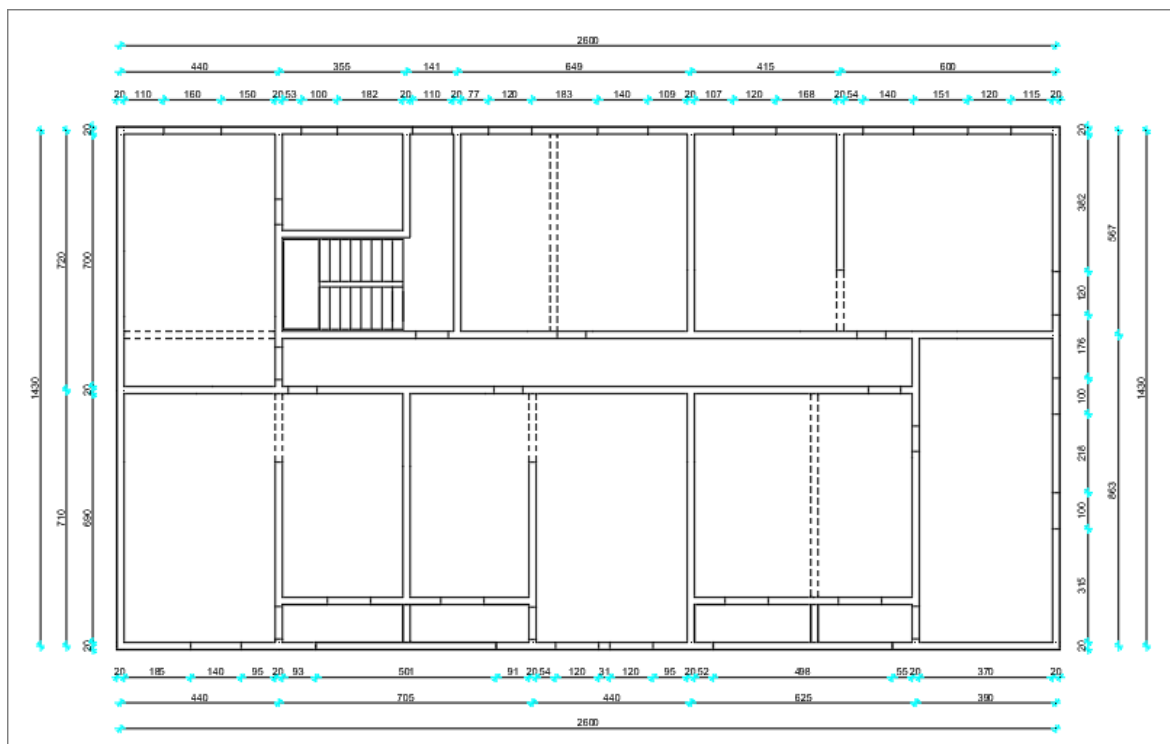
Slika 2. Karakteristični tlocrt
