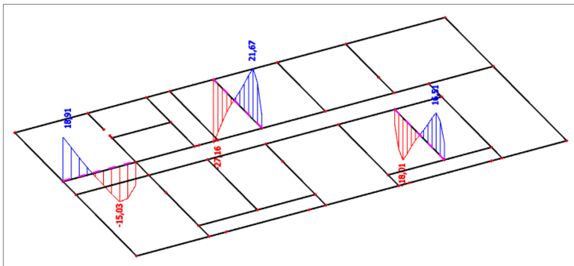
Slika 42. Poprečne sile V_z (kN) za GSN
