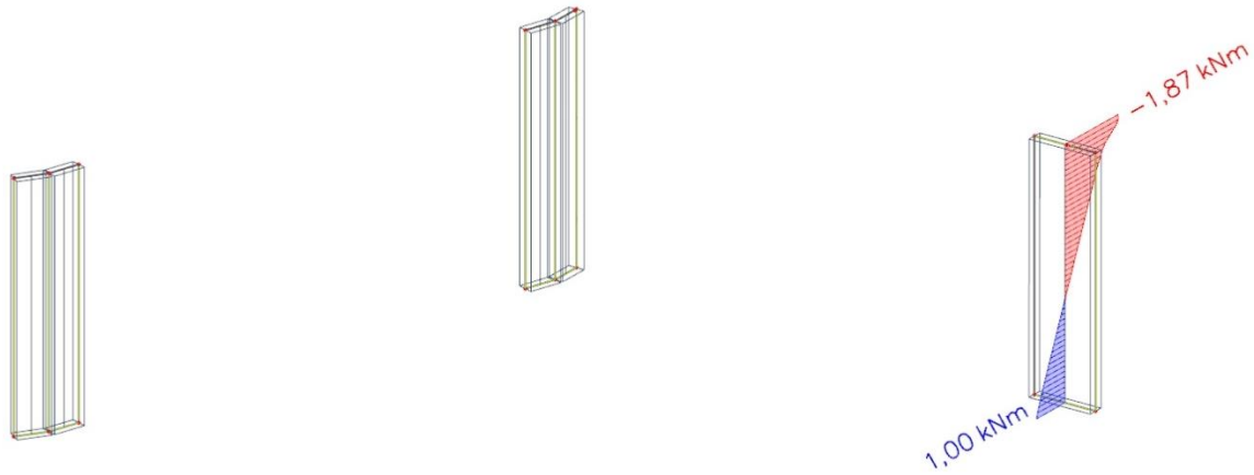
Slika 7.20. M_{z_{\max}} [kNm]
