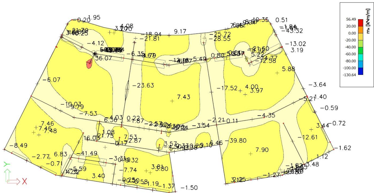
Slika 5.16. Dijagram momenata savijanja M_x [kNm/m']
