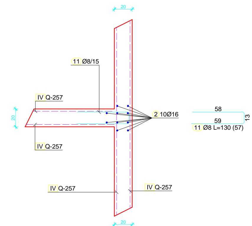
Presjek 2 - 2 (spoj zidova) M 1:25
