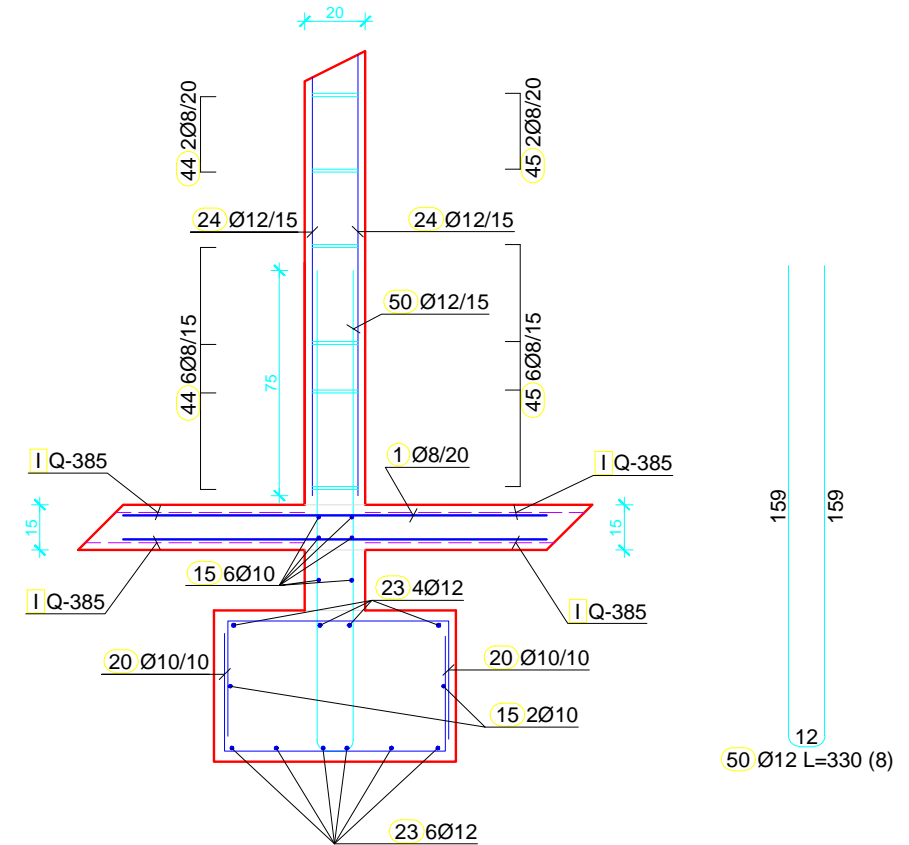
Presjek 2 kroz temelj samac
