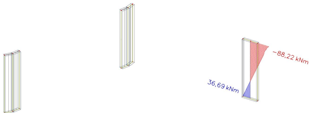
Slika 7.18. M_{y_{\text{prip}}} [kNm]
