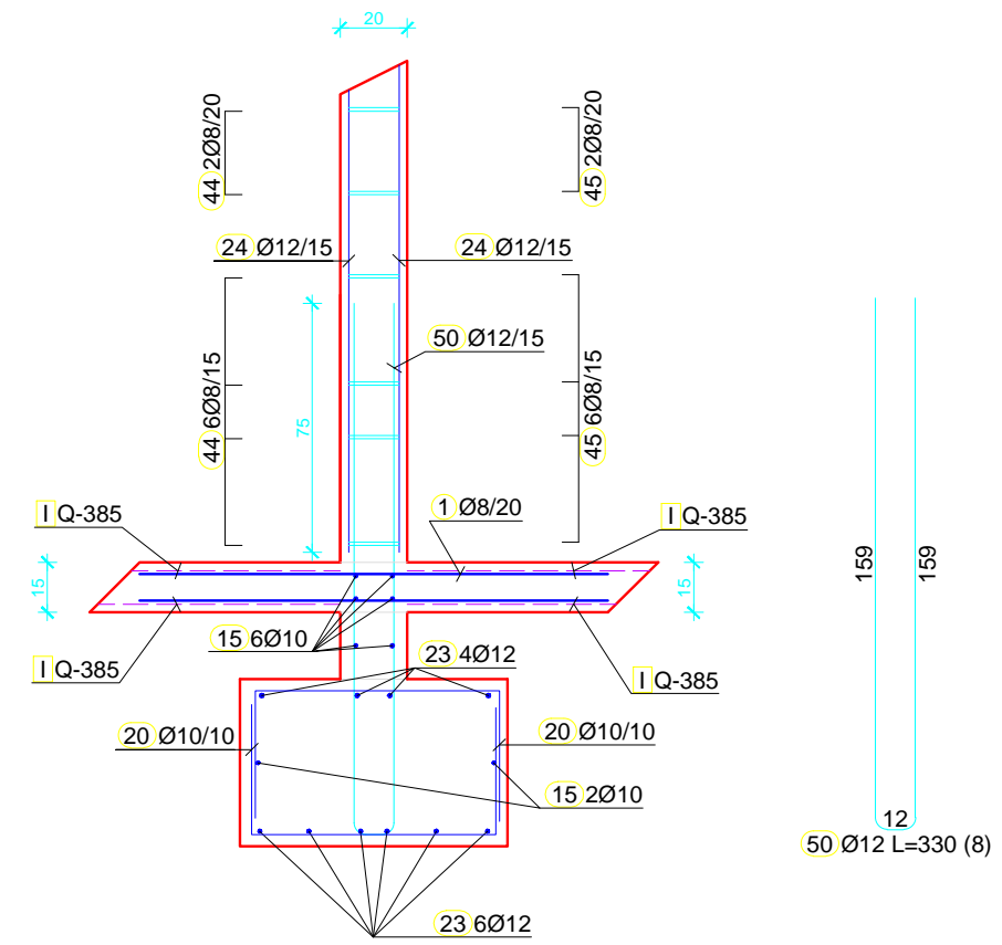
Presjek 2 kroz temelj samac
