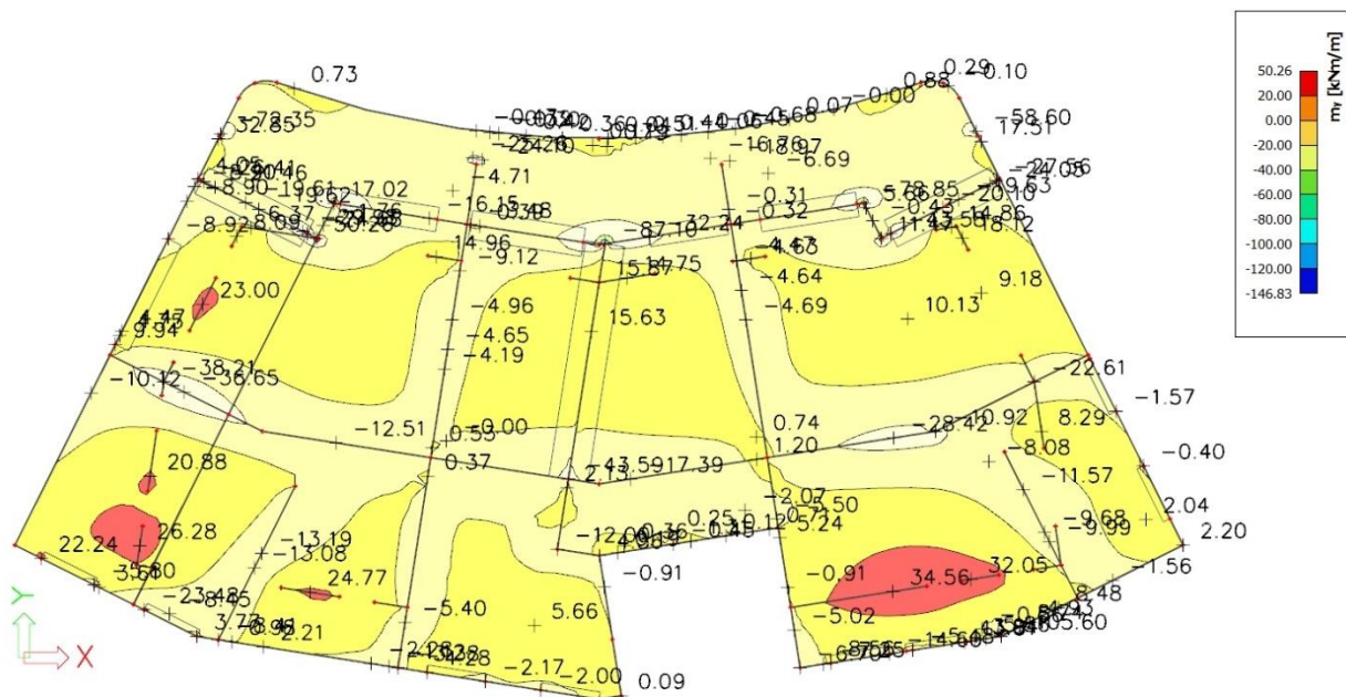
Slika 5.11. Dijagram momenata savijanja M_y [ \text{kNm/m} ']
