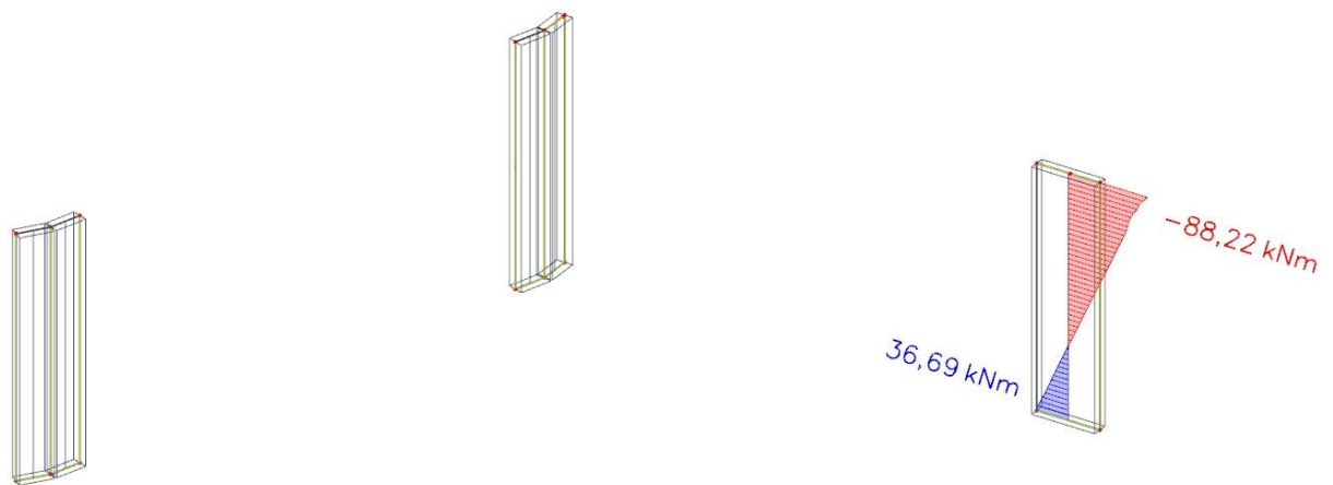
Slika 7.18. M_{y_{\text{prip}}} [kNm]
