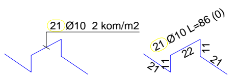
Jahači za gornju zonu M 1:25
