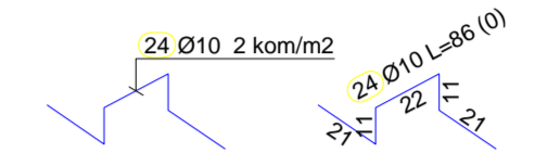
Jahači za gornju zonu M 1:25
