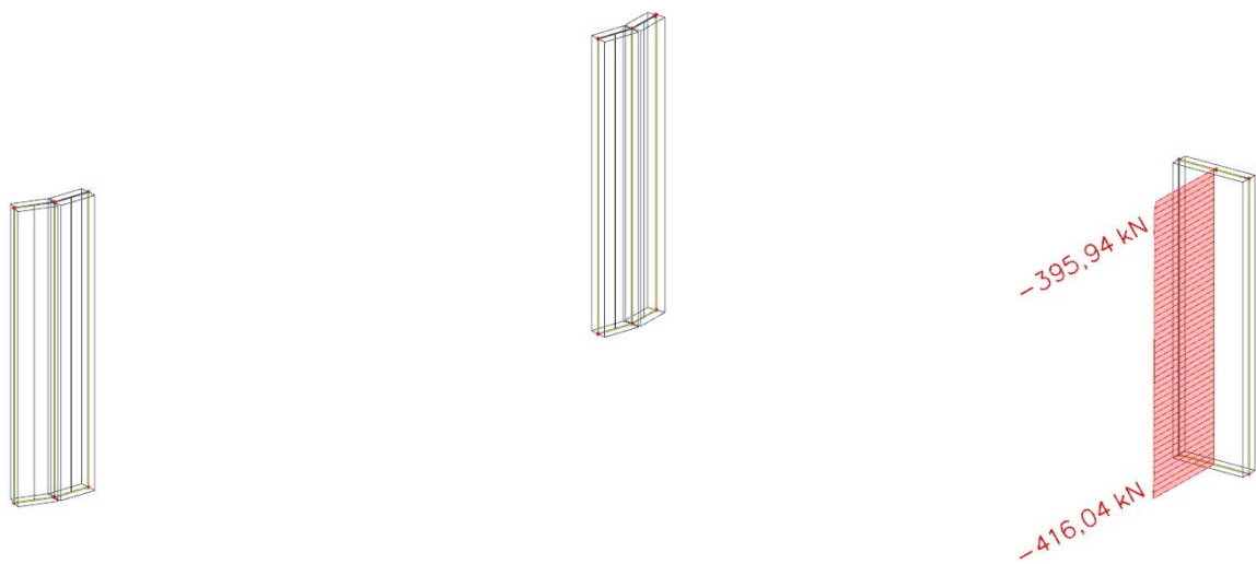
Slika 7.21. N_{\text{prip}} [kN]
