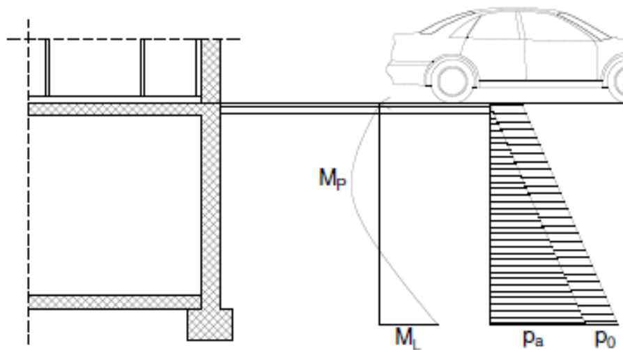
Slika 7.10. Prikaz opterećenja na obodni zid garaže
