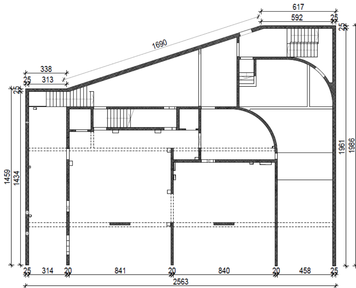
Slika 1.7 Tlocrt razine -1
