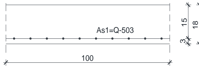
Slika 10.14 Skica armature ploče u polju
