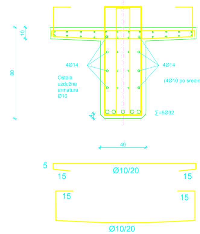
Presjek 2-2
