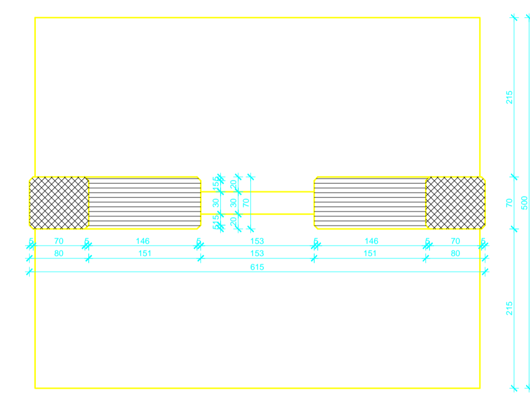
Presjek 3-3
