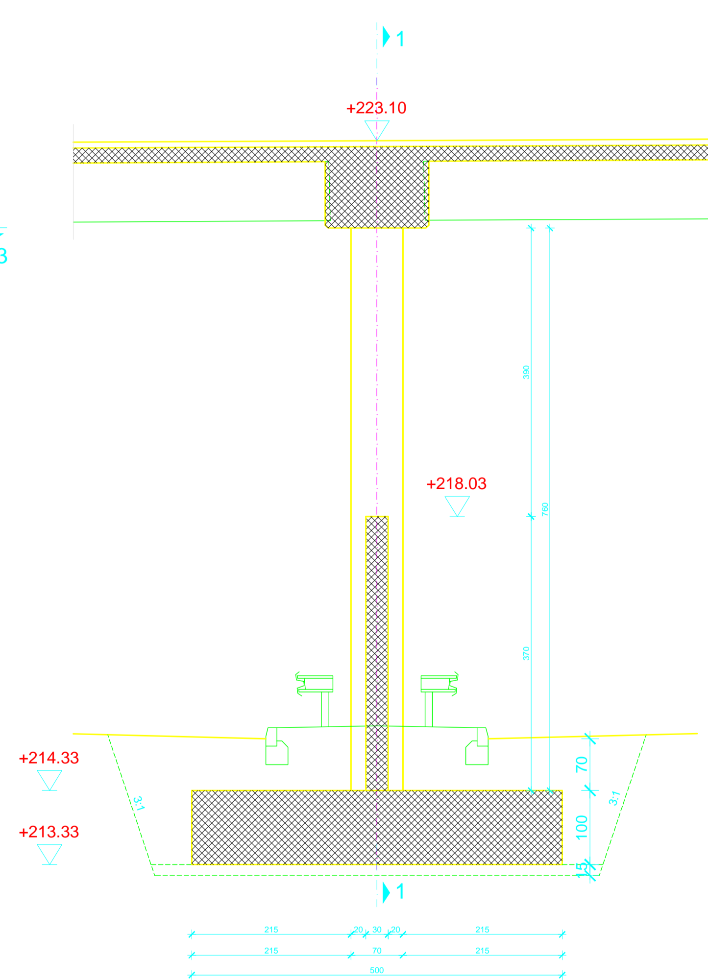
Presjek 2-2
