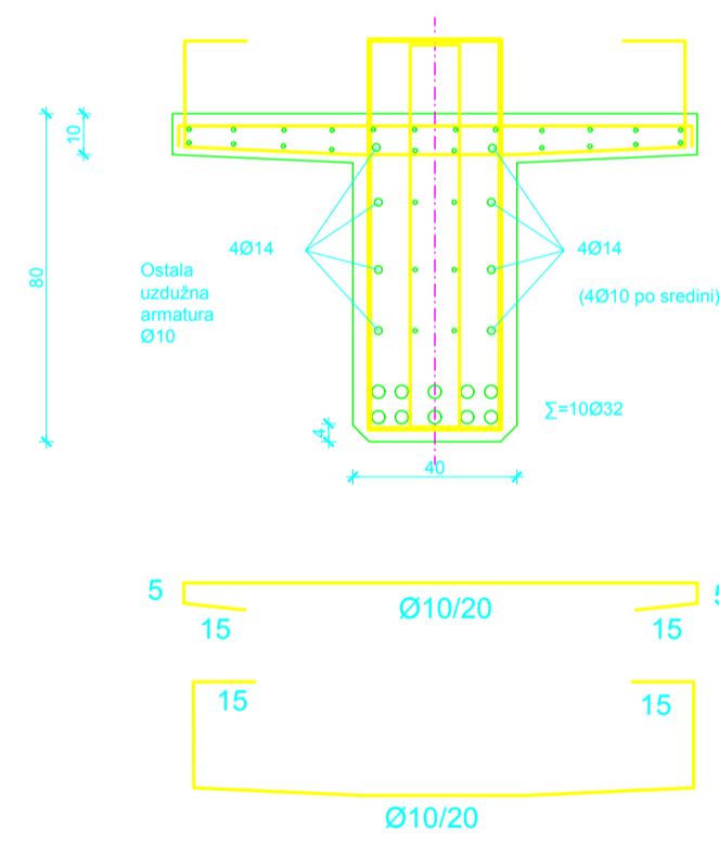
Presjek 1-1
