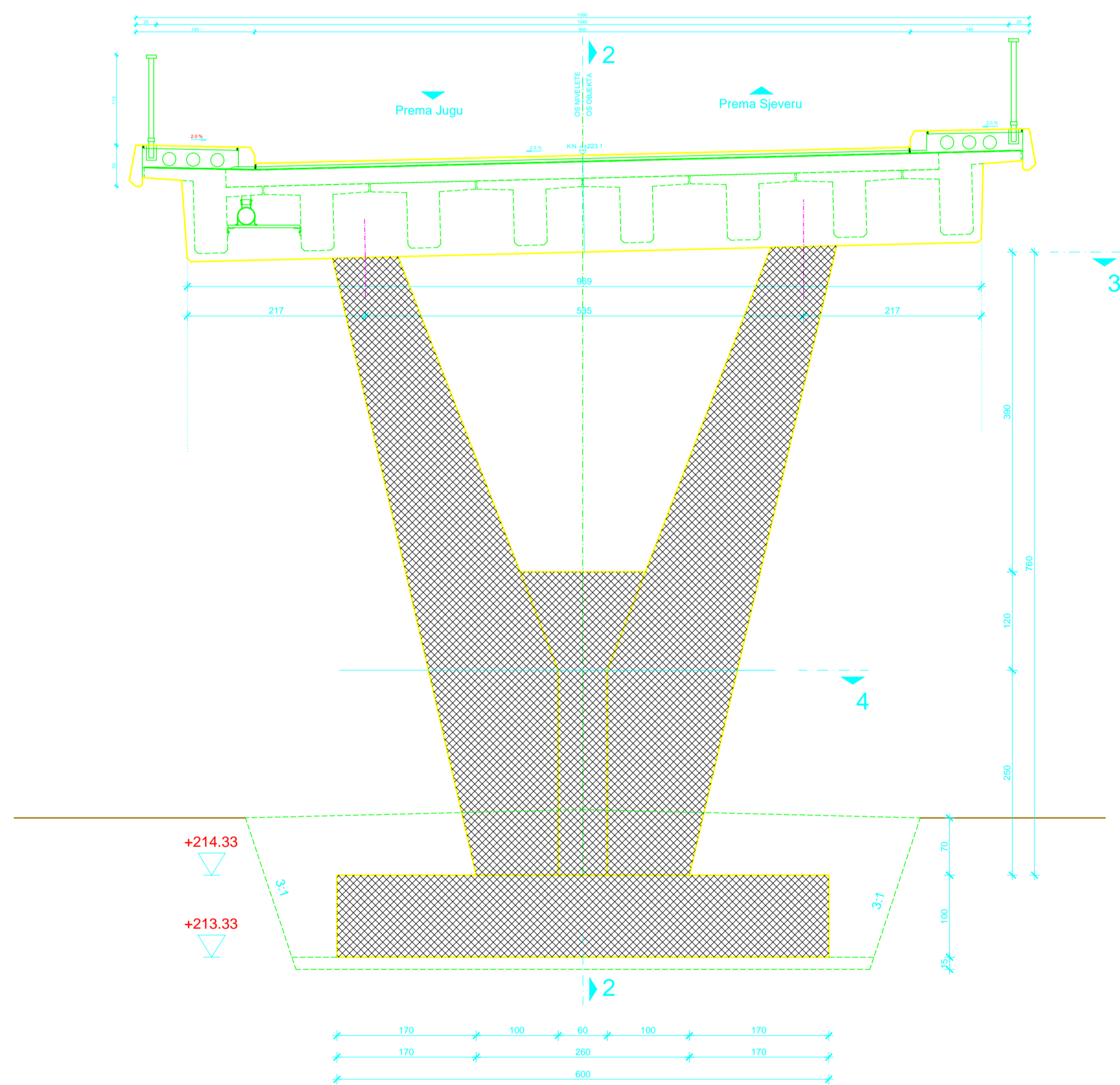
Presjek 1-1
