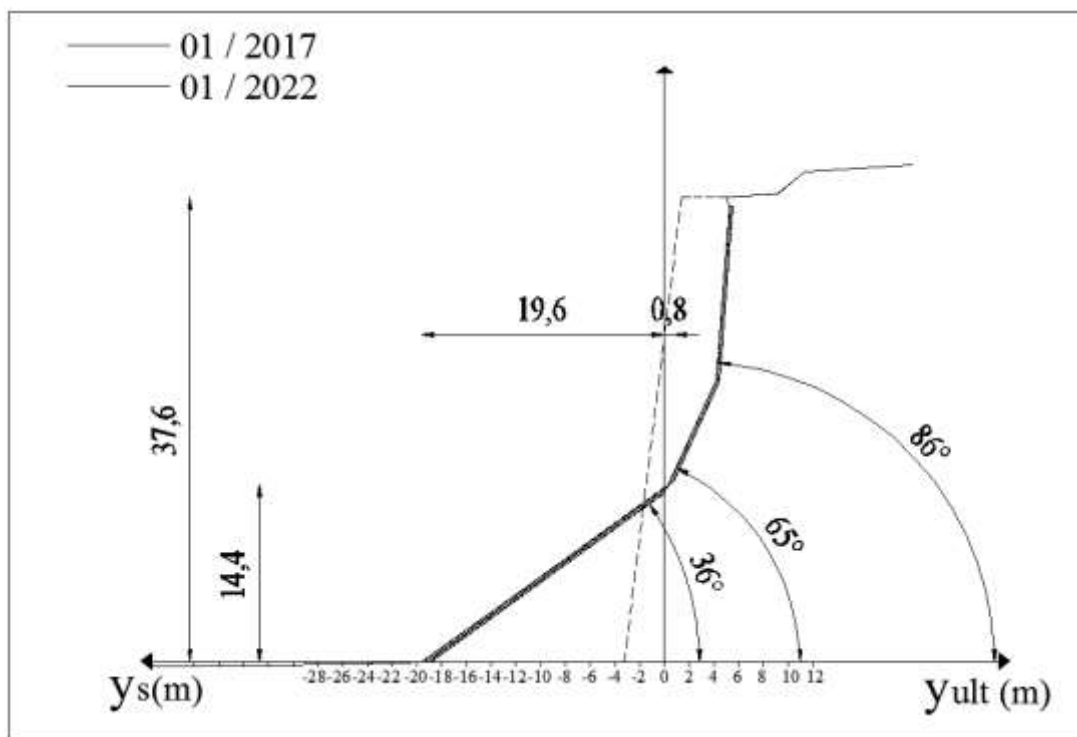
Slika 13. Trenutno lice zasjeka, \Delta T=0 god.
