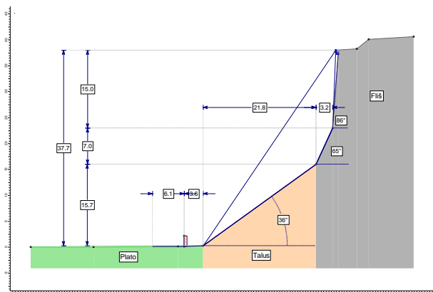
(a) Geometrija zaszjeka sa barijerom h=2 m
