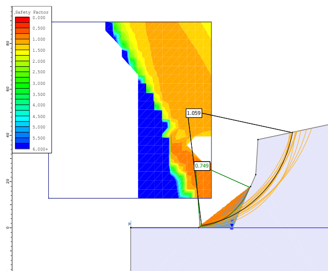
Slika 43. Analiza globalne sigurnosti kosine za \Delta T=20 god.
