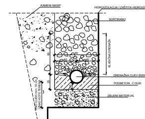
DETALJ DRENAŽE
