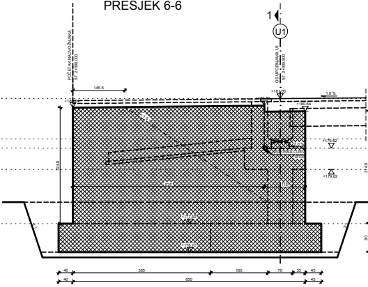
PRESJEK 6-6
