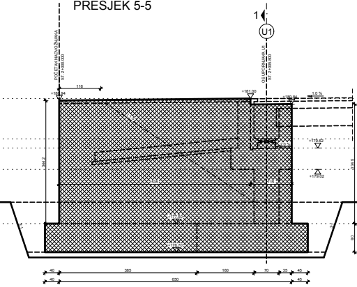
PRESJEK 5-5
