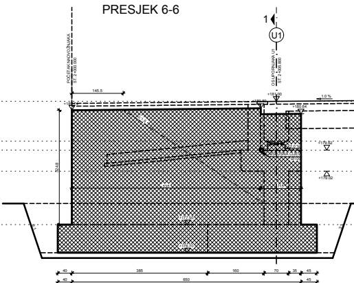
PRESJEK 6-6
