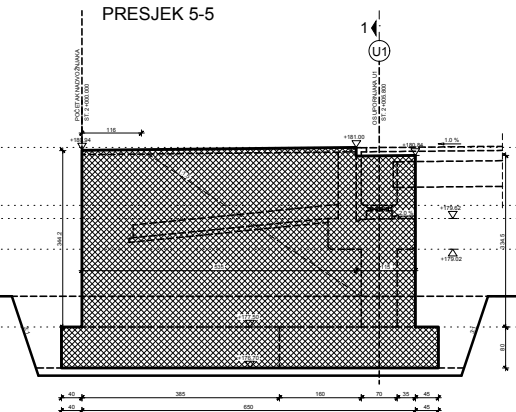
PRESJEK 5-5
