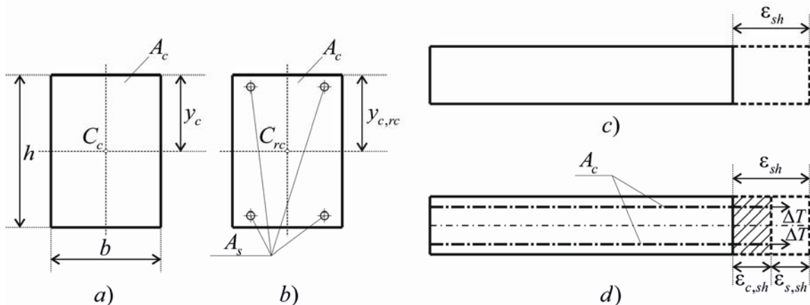
Crtež 4.3. a) Betonski nearchmirani poprečni presjek, b) simetrični armiranobetonski poprečni presjek, c) deformacija skupljanja kod nearchmiranog presjeka i d) deformacija skupljanja kod simetrično armiranog presjeka [G.12]
