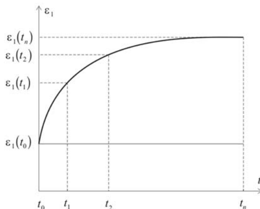
Crtež 4.15. Deformacija puzanja u glavnom pravcu 1 [K.3]
