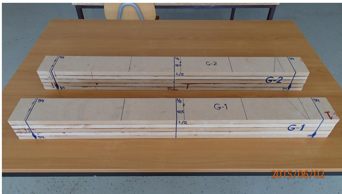
Fotografija 4.2: Prikaz označavanja grede
