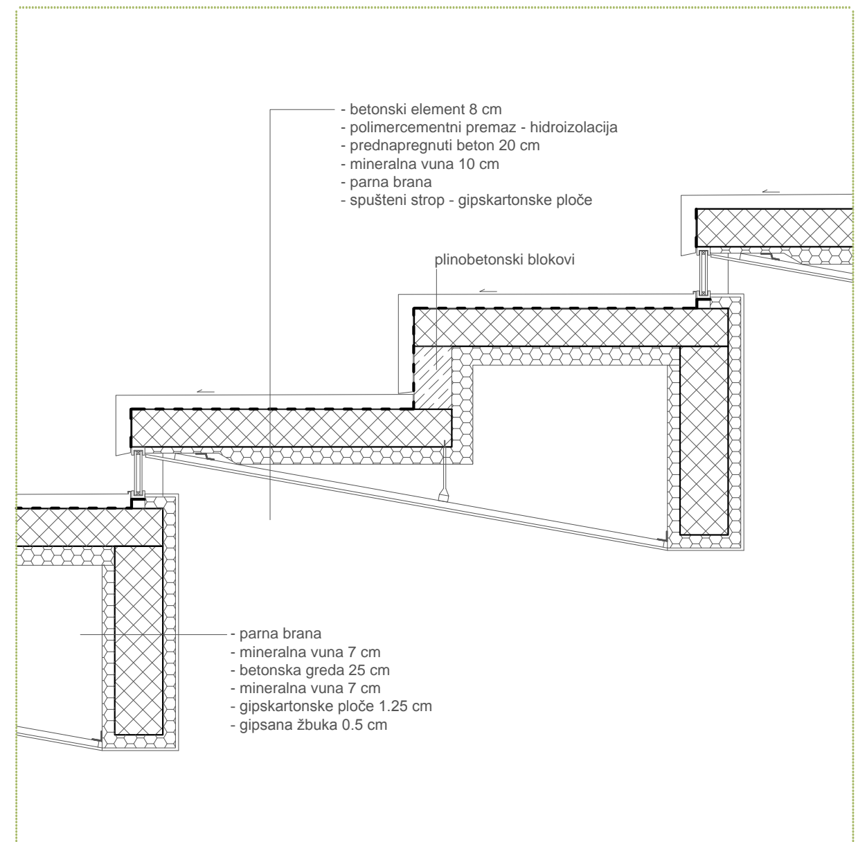
DETALJ TRIBINA
