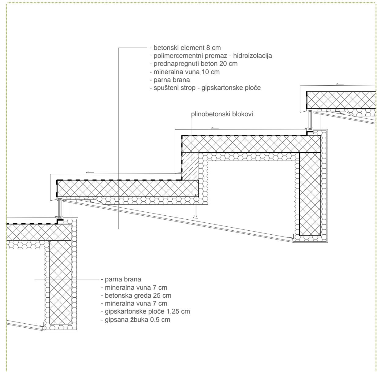
DETALJ TRIBINA
