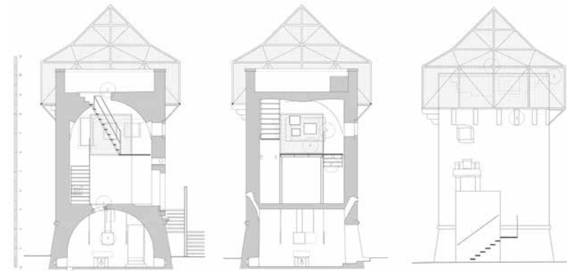
PRESEK 1-1
