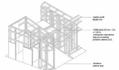
ŠEMATSKI PRIKAZ KONSTRUKCIJE
