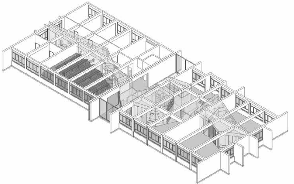
AKSONOMETRIJA
