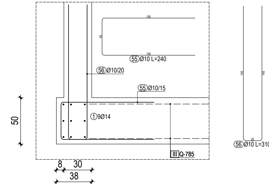
DETALJ 2-2 M 1:25
