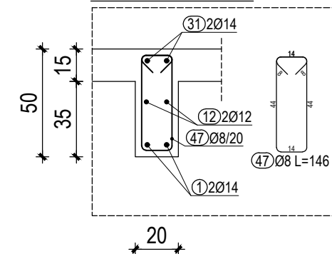
DETALJ 1-1 M 1:25
