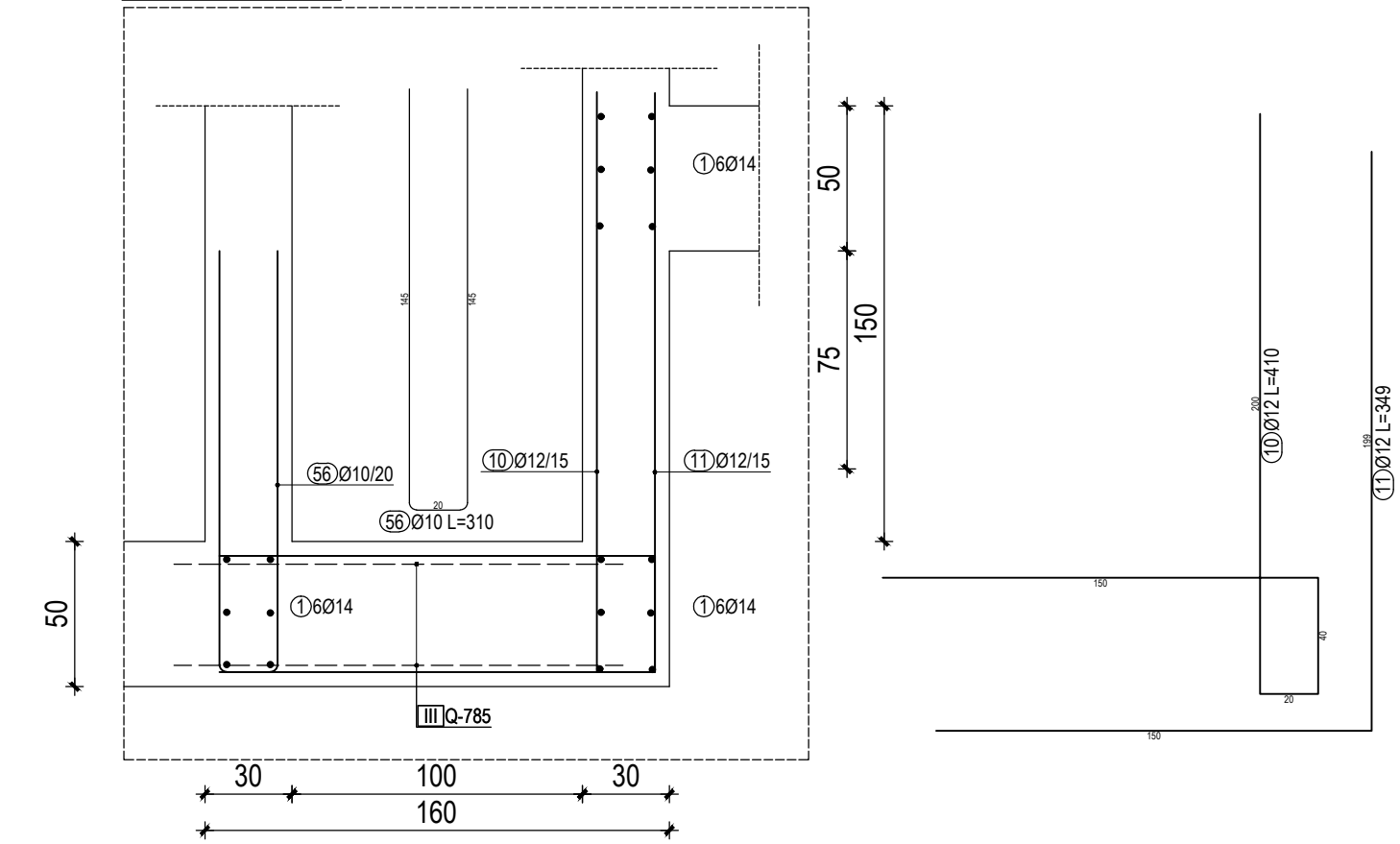
DETALJ 2-2 M 1:25
