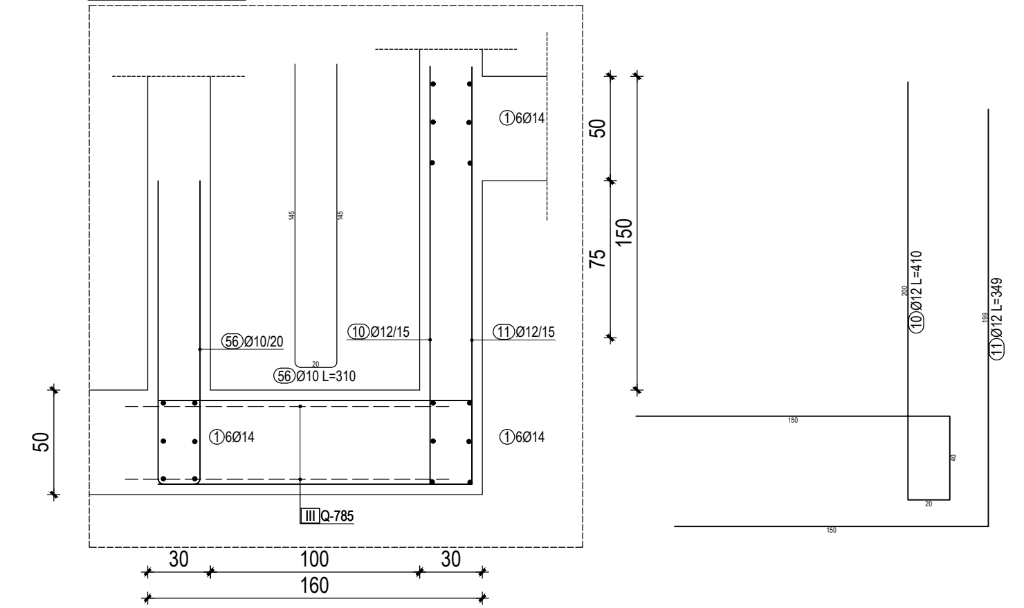
DETALJ 2-2 M 1:25
