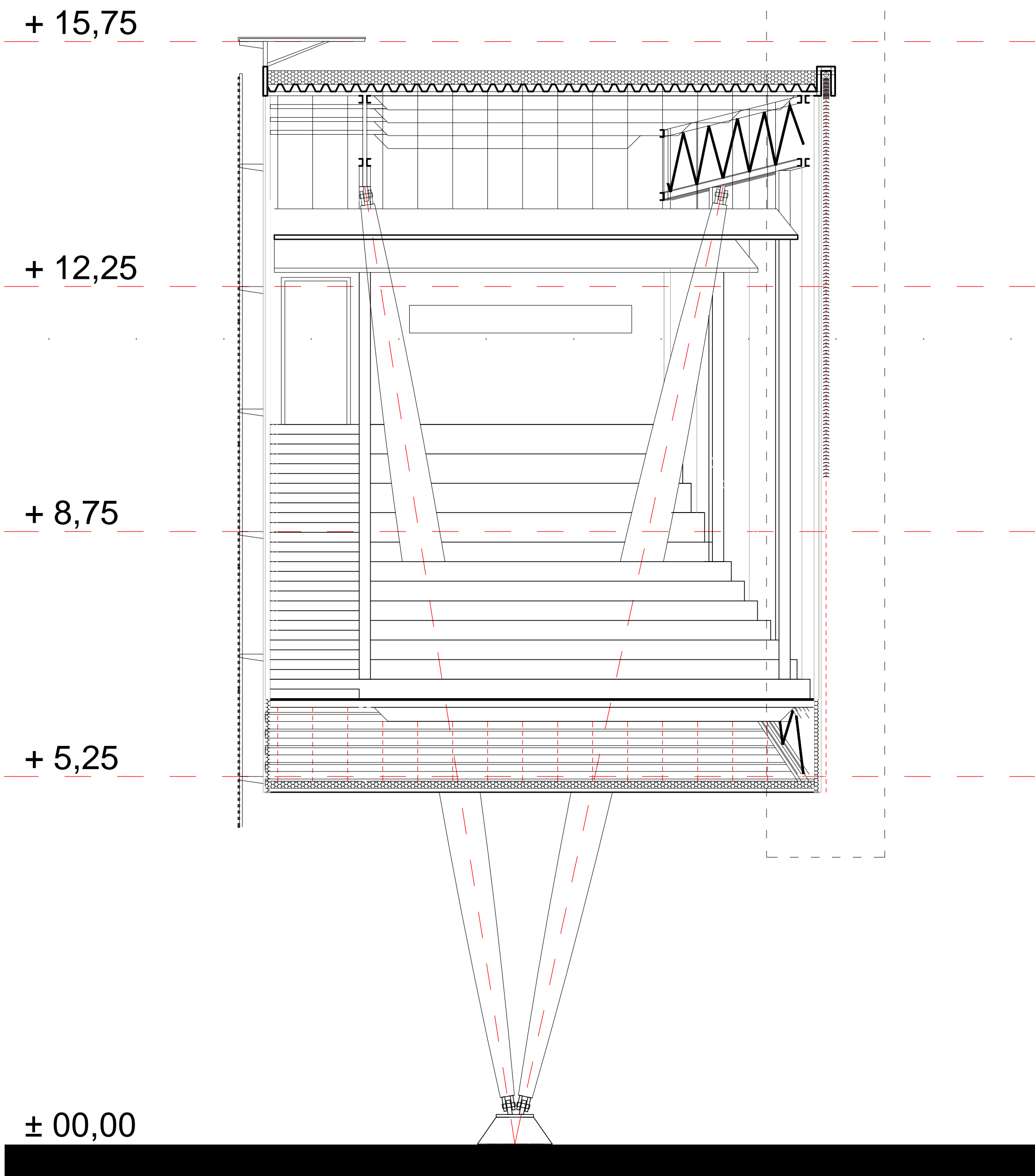
PRESJEK M 1:50
