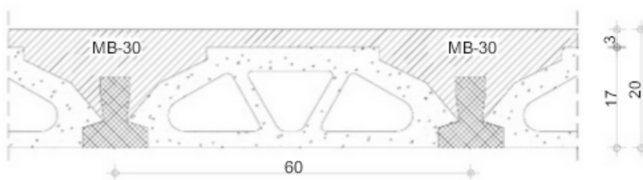
Slika 2.23: Poprečni presjek stropa tipa MK-20 – T6 ili T4
