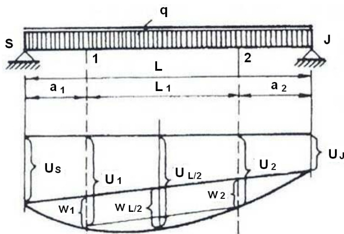
Crtež 4.3: Postupak eliminacije pomaka oslonaca
