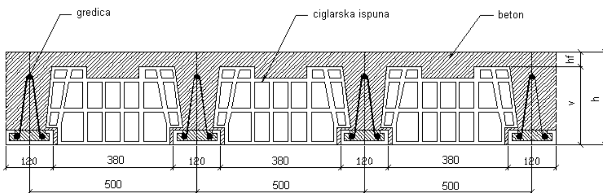
Slika 2.11: Poprečni presjek Fert stropa
