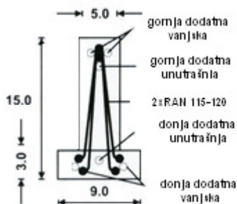
Slika 2.28: Poprečni presjek gredice
