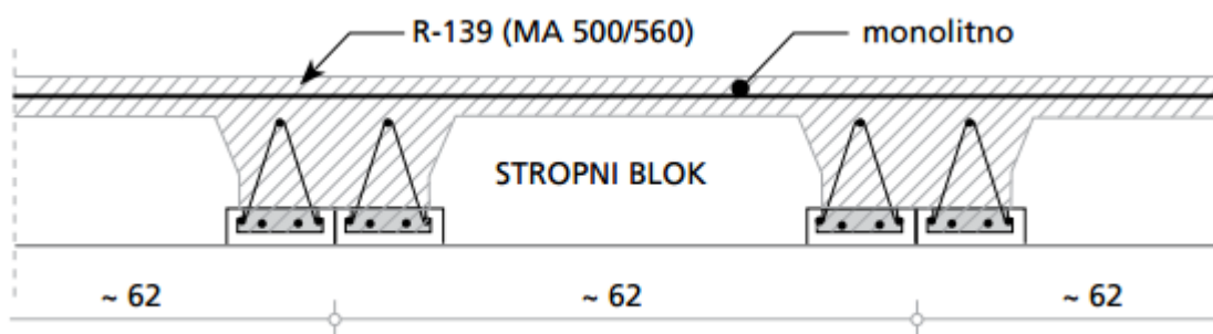
Slika 2.18: Strop s udvojenim gredicama
