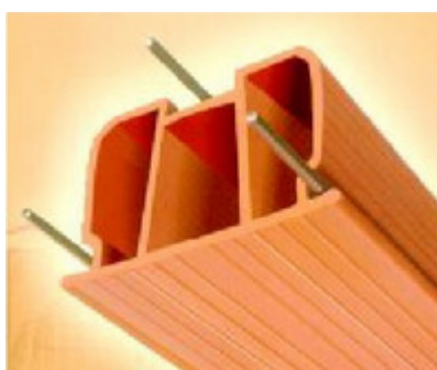
Slika 2.9: Monta opeka s umetnutom armaturom
