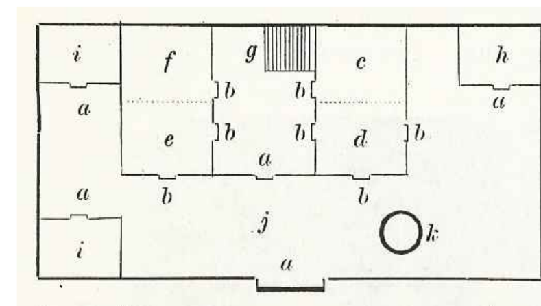
Grafički prilog 43. POJATA
