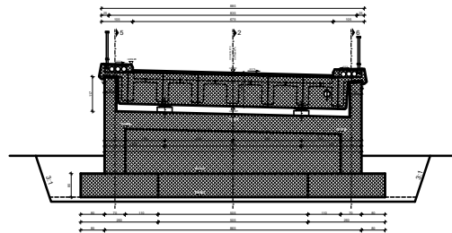
PRESJEK 1-1
