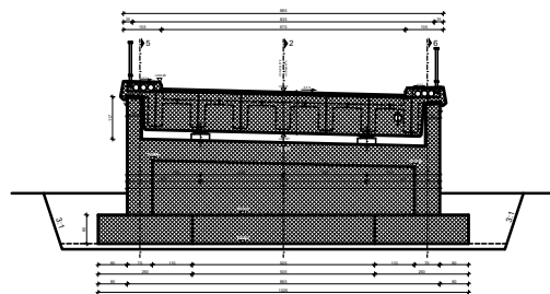
PRESJEK 1-1
