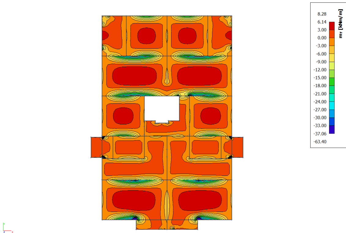
Slika 6.27. Dijagram momenata savijanja M_y [kNm/m']
