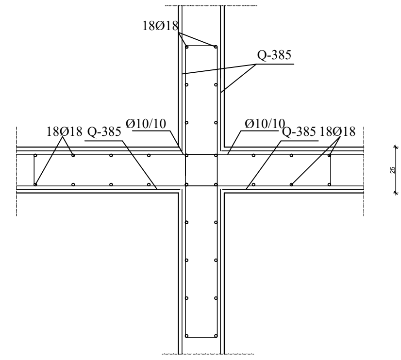
Detalj C
