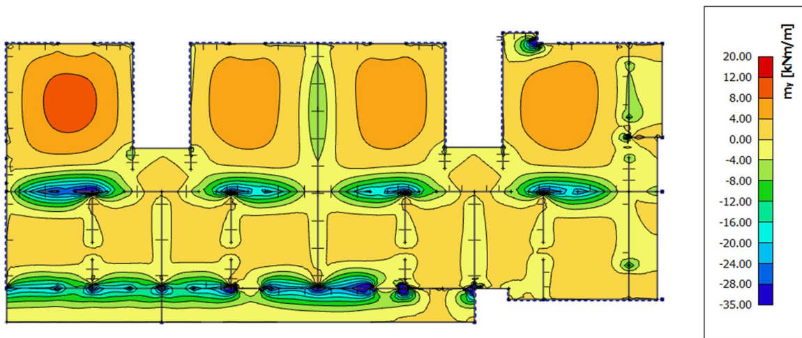
Slika 11.12 Prikaz momenata savijanja – m_y
