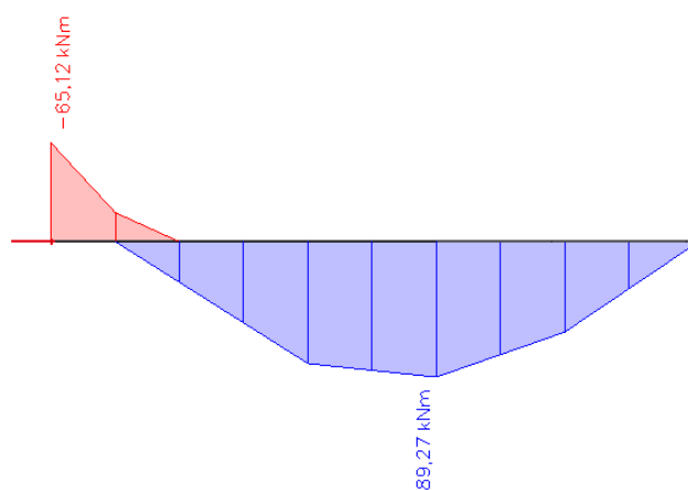
Slika 11.1 Maksimalni momenti savijanja M_y
