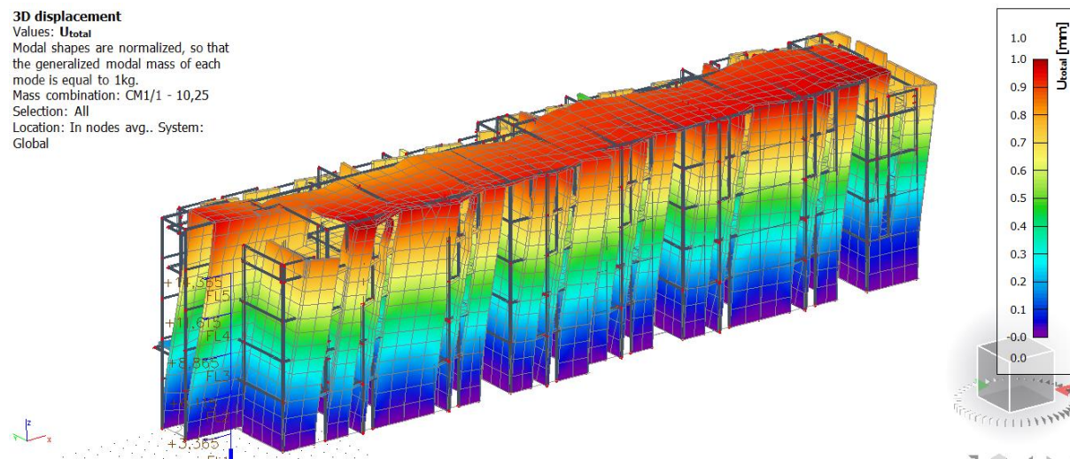
Slika 9.2 1.mod translacija u smjeru globalne osi x
