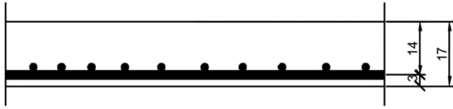
Slika 10.29 Skica armature ploče u polju
