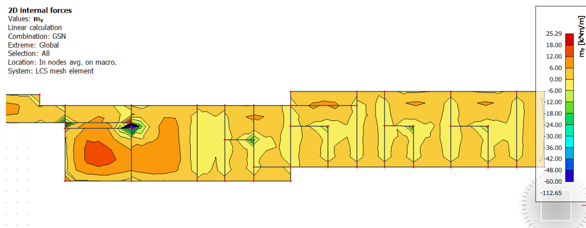
Slika 10.3 Prikaz momenaza savijanja (GSN, m_y )
