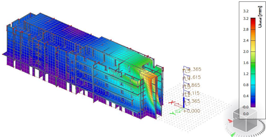
Slika 9.3 2. mod translacija u smjeru globalne osi y
