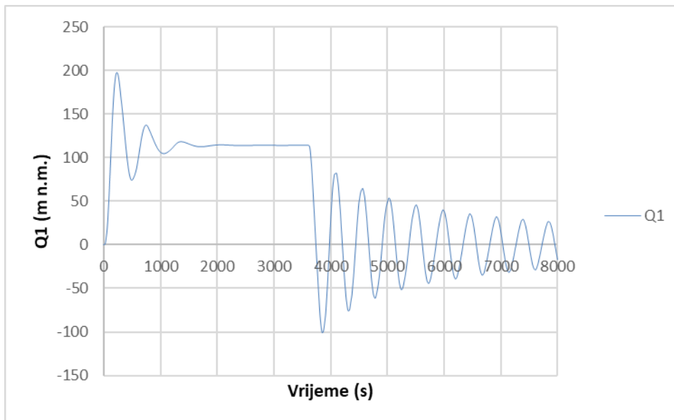
Slika 36 Protok Q1 u ovisnosti o vremenu za Varijantu 1.2
