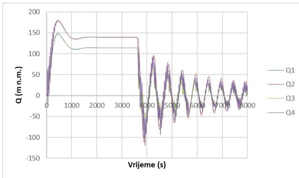
Slika 150 Protoci u dovodnim tunnelima 1, 2, 3 i 4 u ovisnosti o vremenu za Varijantu 7.1
