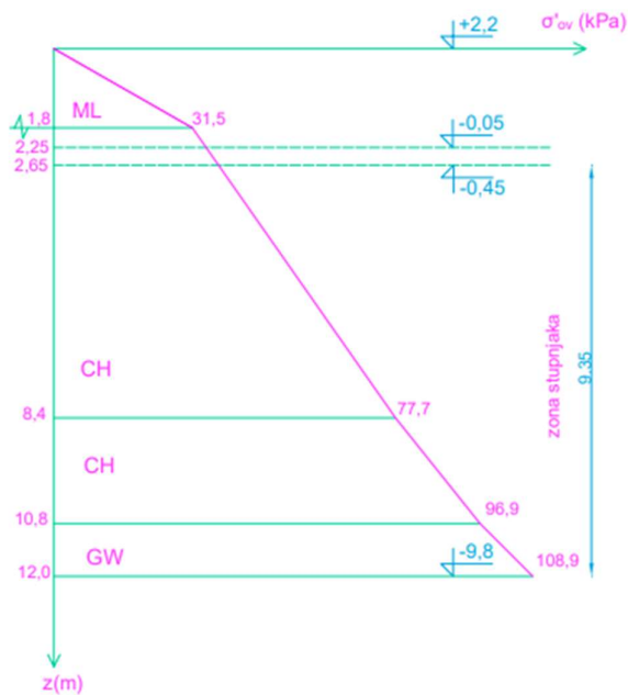
Slika 4: Prikaz pripadajućeg dijagrama vertikalnog efektivnog naprezanja za B – 1
