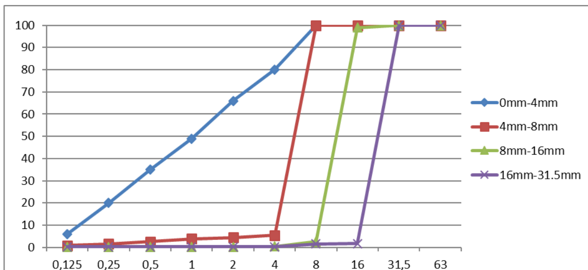
Slika 6.3 Granulometrijske krivulje pojedinih frakcija (Tablica 6.1)
