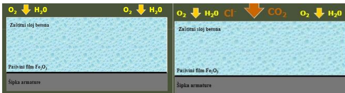
Slika 2.7 Pasivizacija (lijevo), Depasivizacija (desno)
