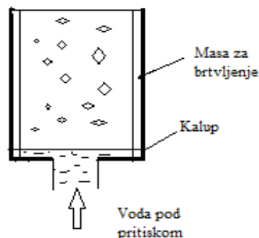
Slika 5.1 Shematski prikaz ispitivanja vodo-nepropusnosti betona sa spriječenim izlazom vode na bočnim stranama ispitnog tijela
