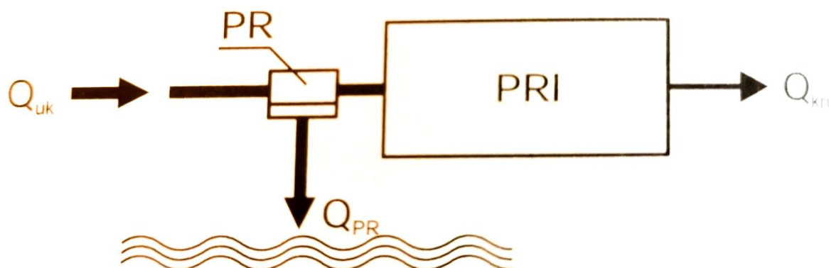
Slika 3. Kišni bazen za prihvat prvog pljuska na glavnom kanalu
