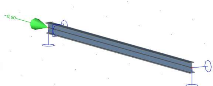
Slika 35 Model krovne podrožnice za djelovanje uzdužne sile.
