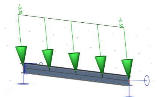
Slika 34 Model krovne podrožnice za djelovanje pritiskajućeg vjetra
