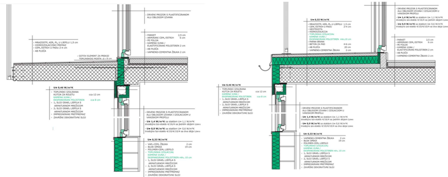
Način rješavanja problema toplinskih mostova kod konzolnih istaka, izvor EIHP
