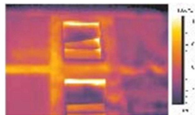
Primjer toplinskog mosta snimljen termografskom kamerom Izvor: EIHP
