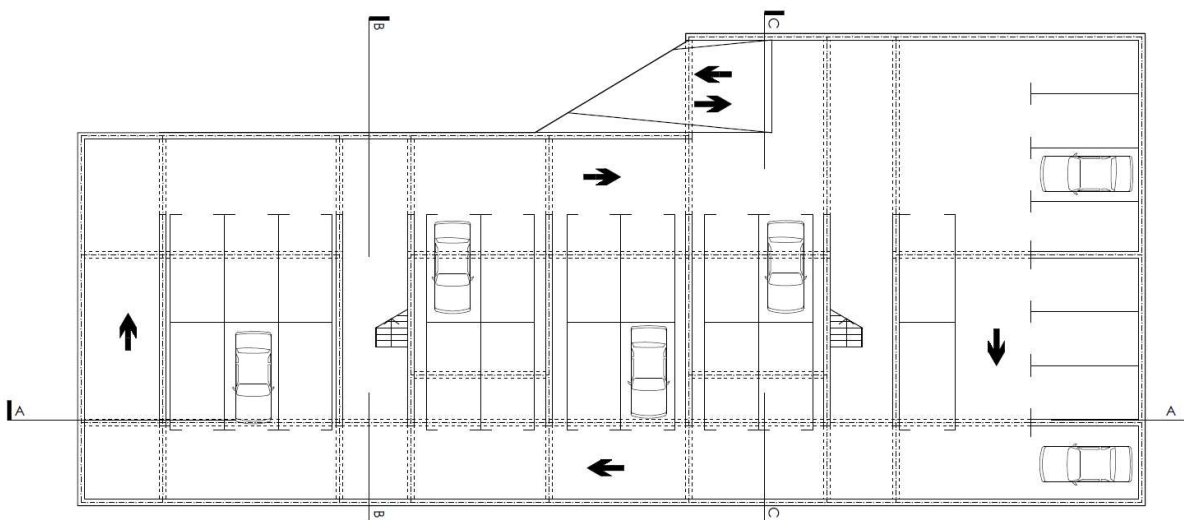
Slika 1.8. Tlocrt garaže
