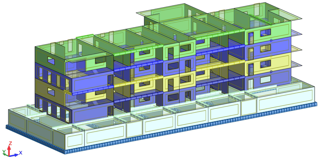
Slika 9.3. 3D model promatranog objekta (3)
