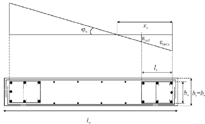
Slika 13.13. Shema potresne armature
