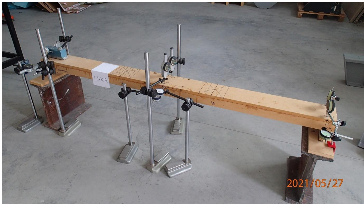
Slika 39: Prikaz grednog nosača nakon montirane cjelokupne opreme za mjerenje
