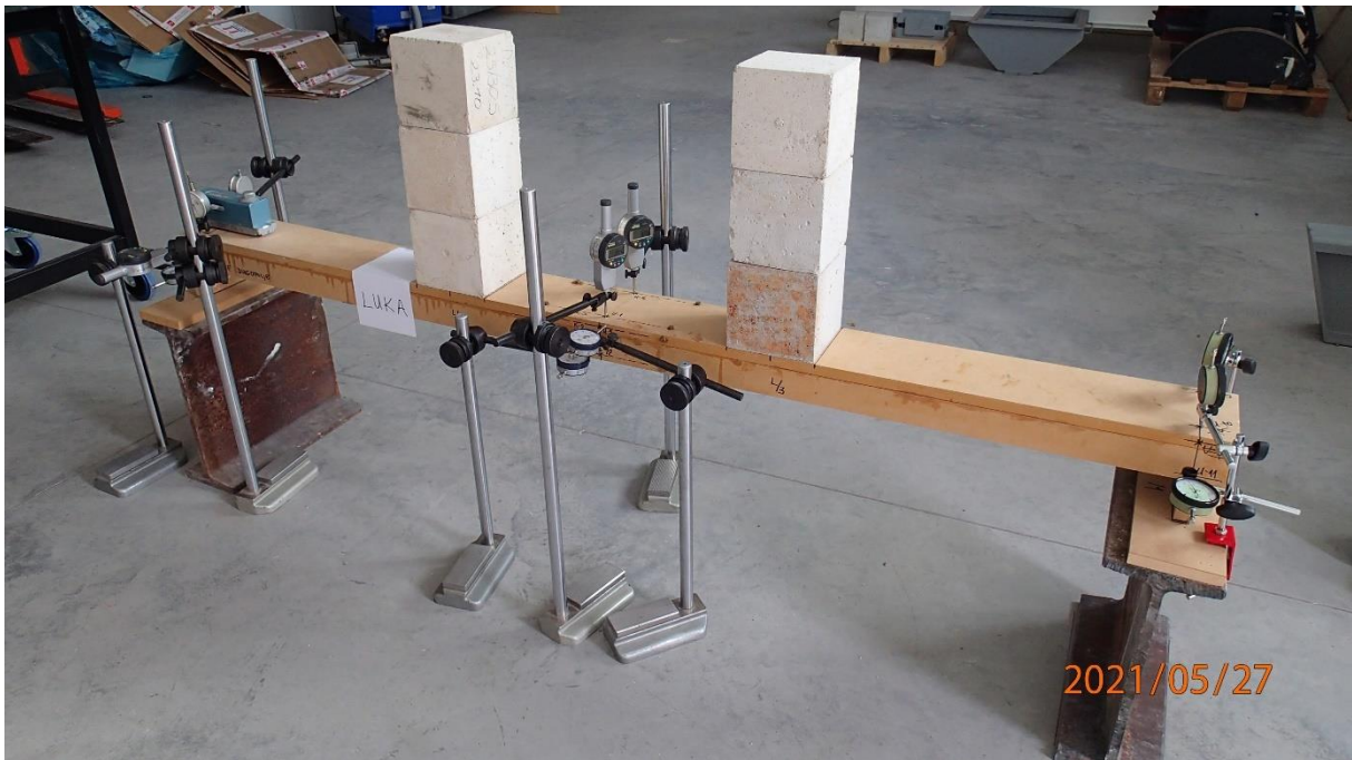
Slika 42: Nosač s tri reda opterećenja, F = 0,24 \text{ kN}
