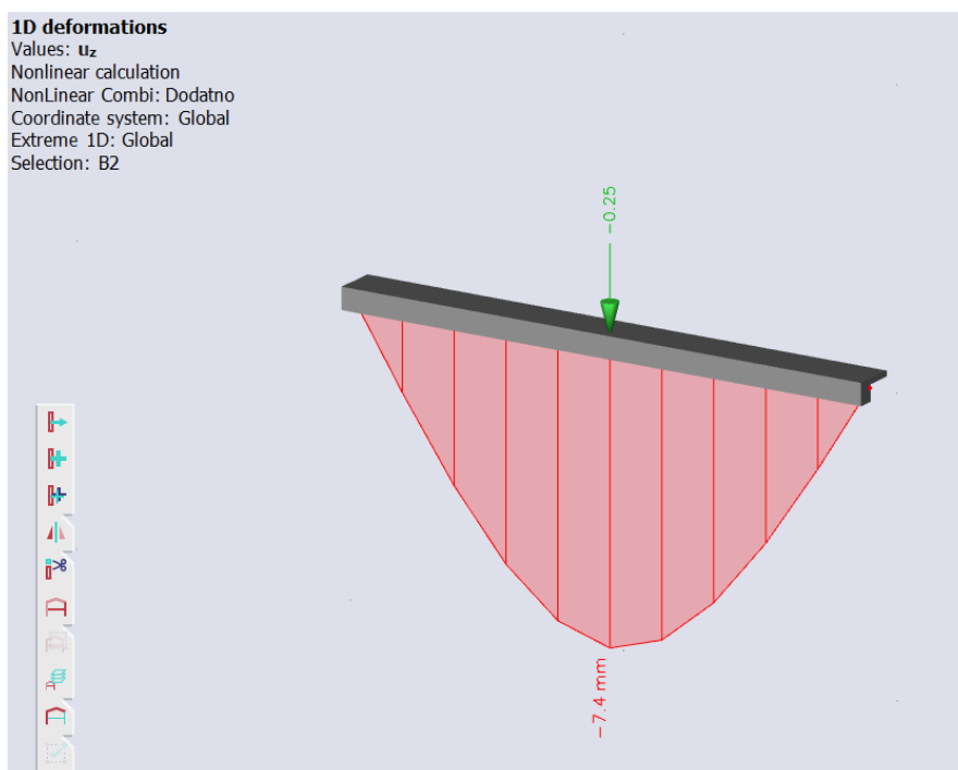
Slika 29: Progib za nelinearni proračun
