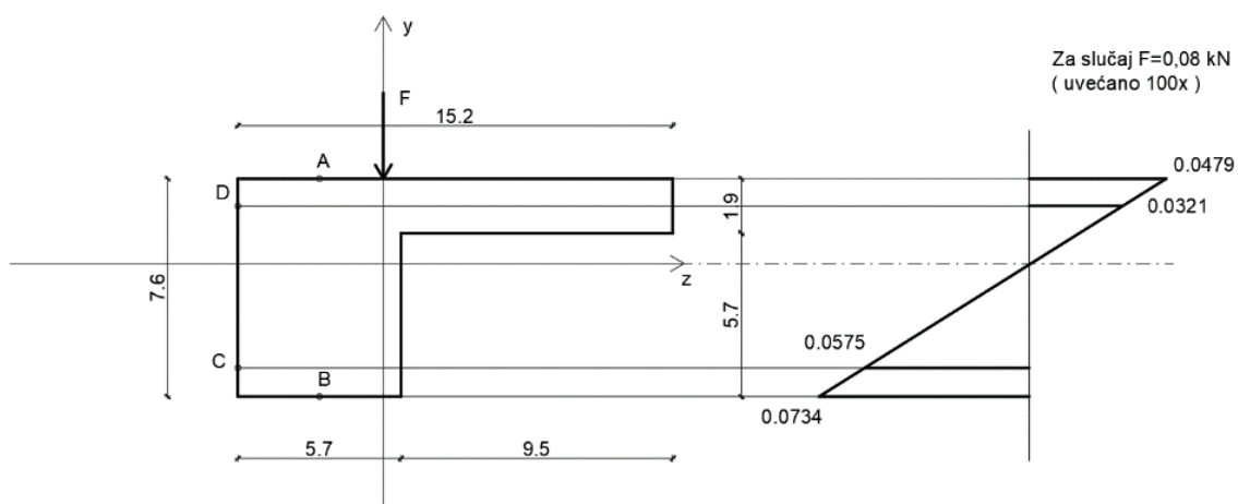
Slika 12: Dijagram naprezanja u slučaju pravog savijanja
